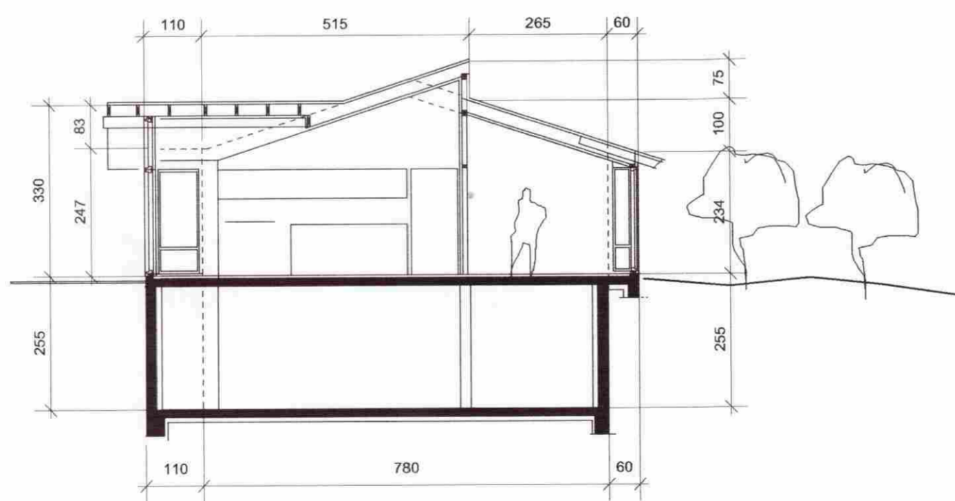
SNEIDING B-B
