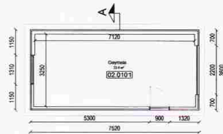
Grunnmynd Mkv 1:100
