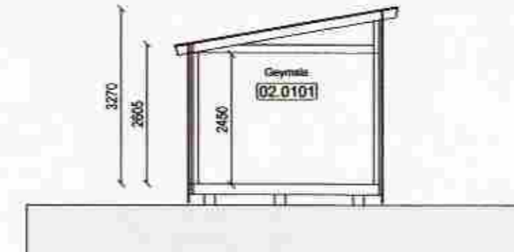
Snið A-A Mkv 1:100
