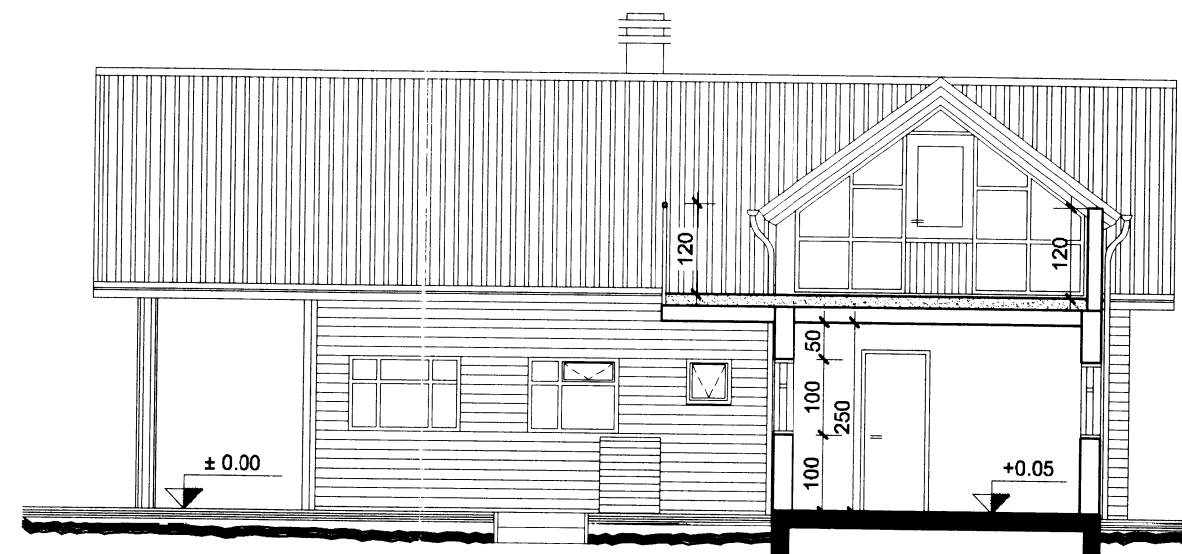
Snið B-B
