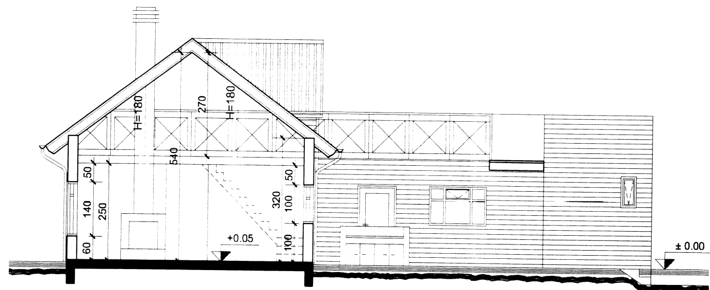
Snið A-A
