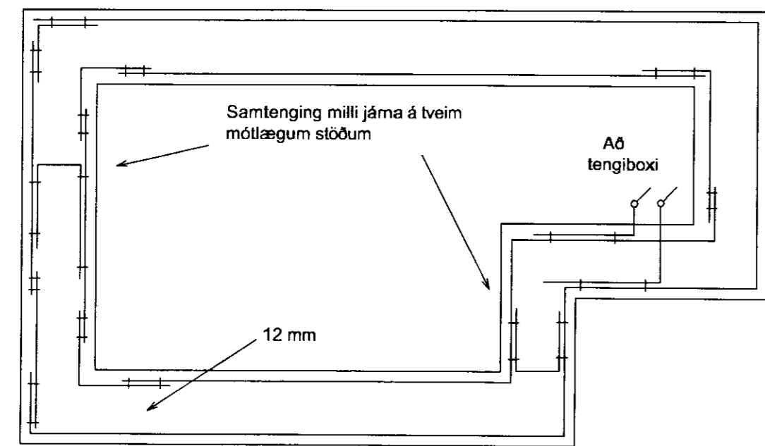
Grundmynd sökkulveggja
