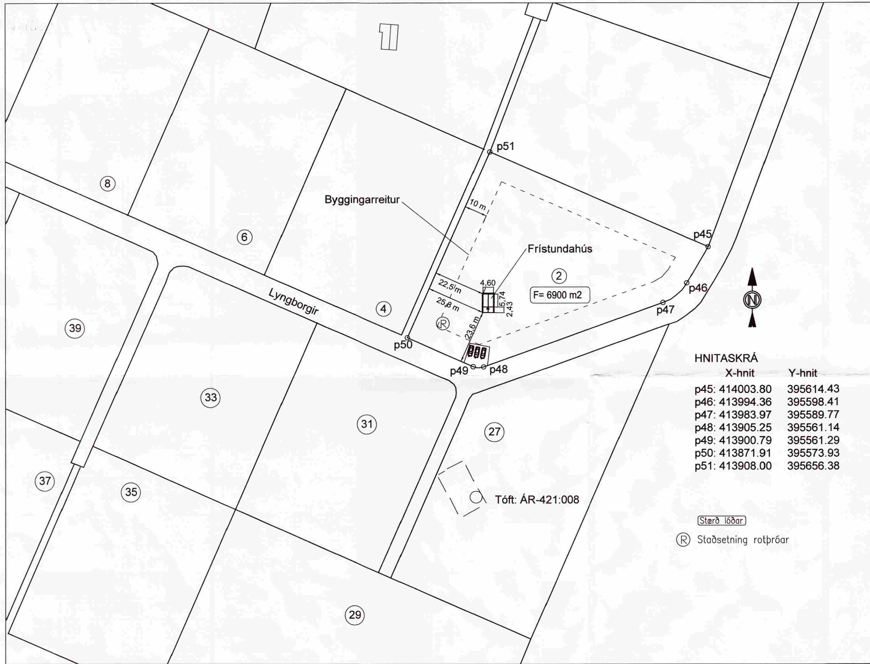
AFSTÖÐUMYND 1:1000
