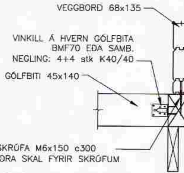
101 SNID MKV. 2
