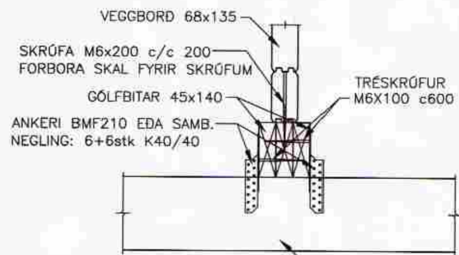
104 SNID MKV. 2
