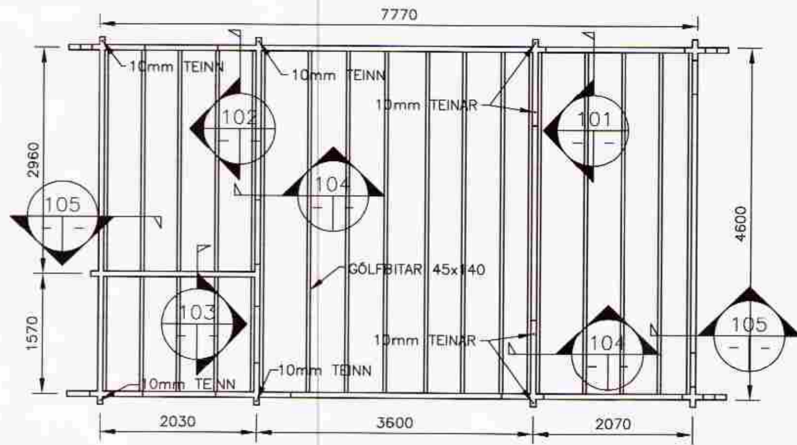
GRUNNMYND-VEGGIR MKV. 1
