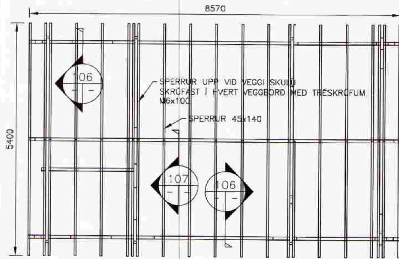
GRUNNMYND-ÞAK MKV. 1
