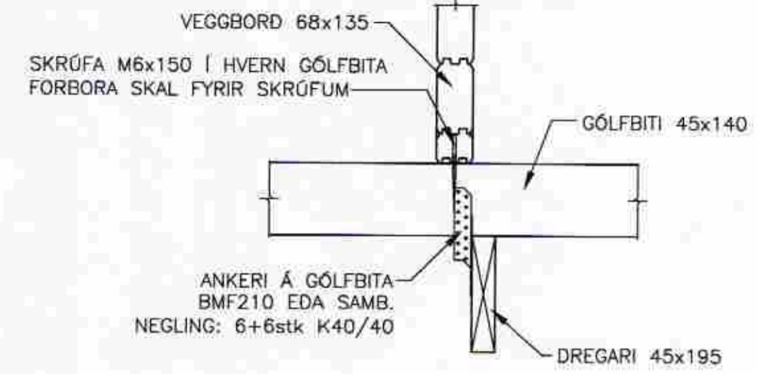
103 SNID MKV. 2
