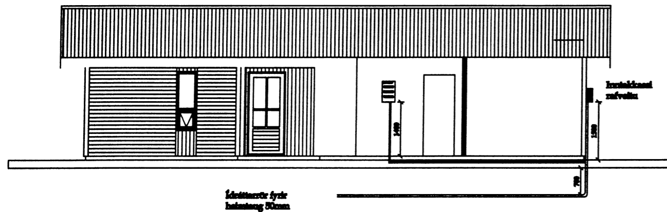
Sniðmynd A-A: 1:50
