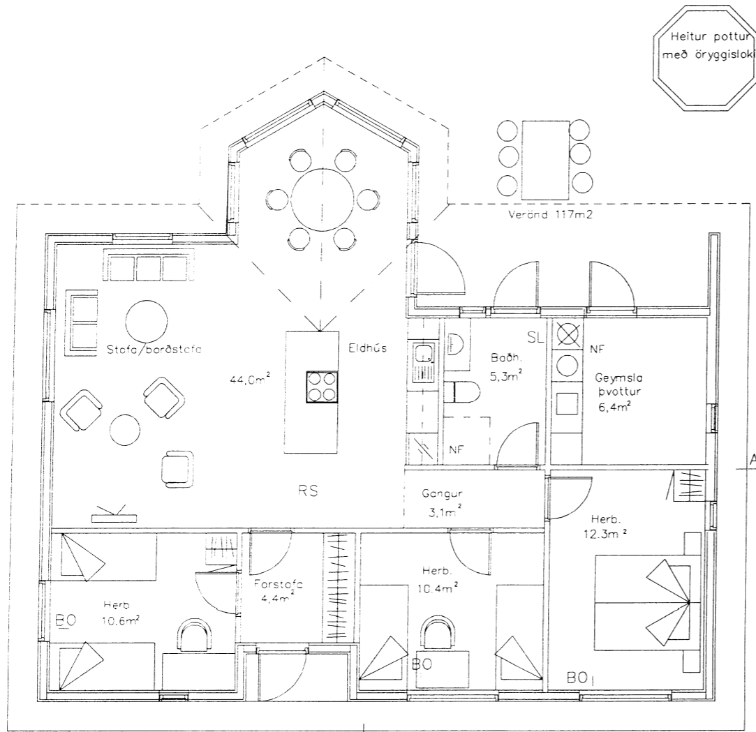
Grunnmynd: 1:50
