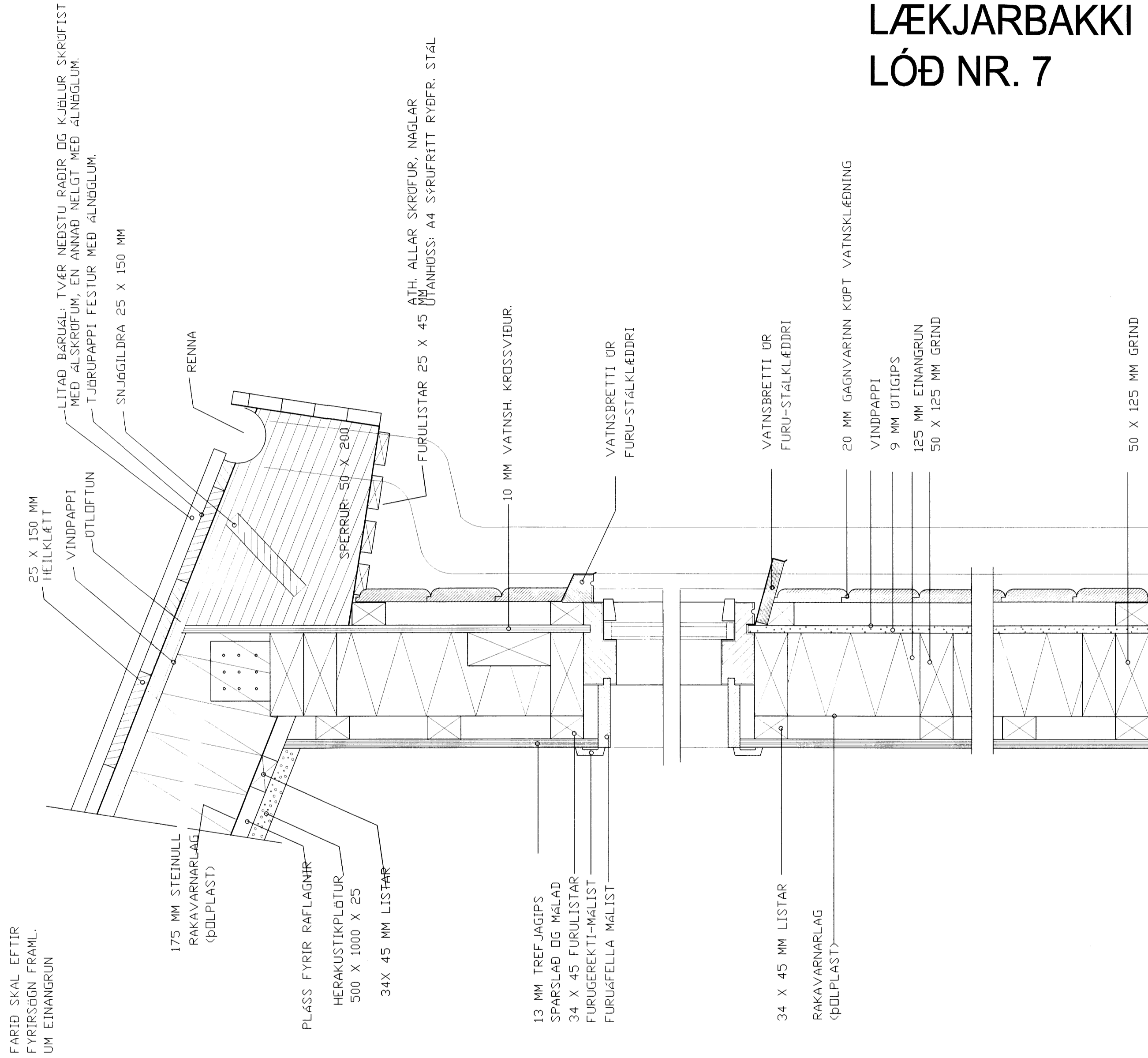
LÓÐRÉTT SNID Í ÚTVEGG OG ÞAK
