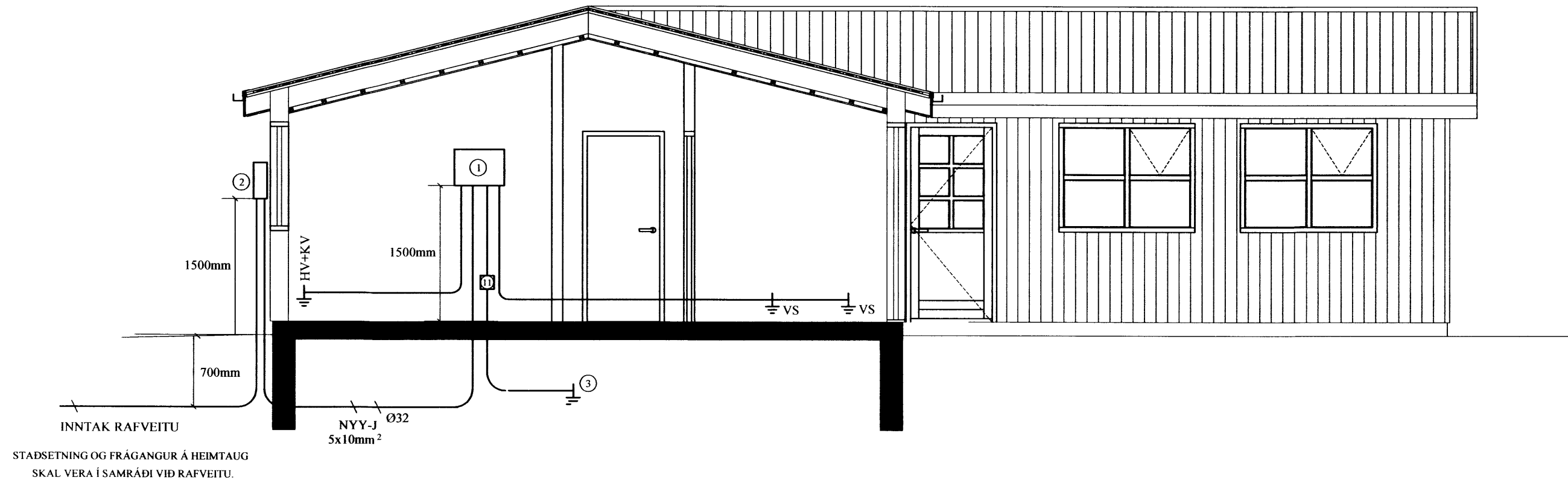
SNID A-A
