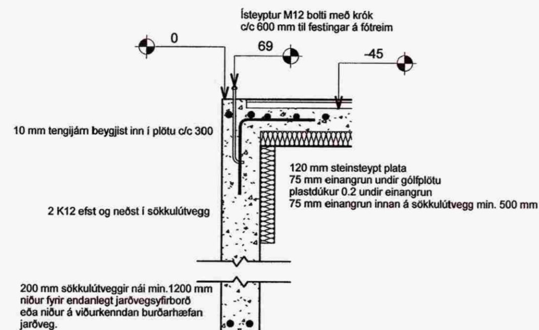
1 Skurður D 1 : 20
