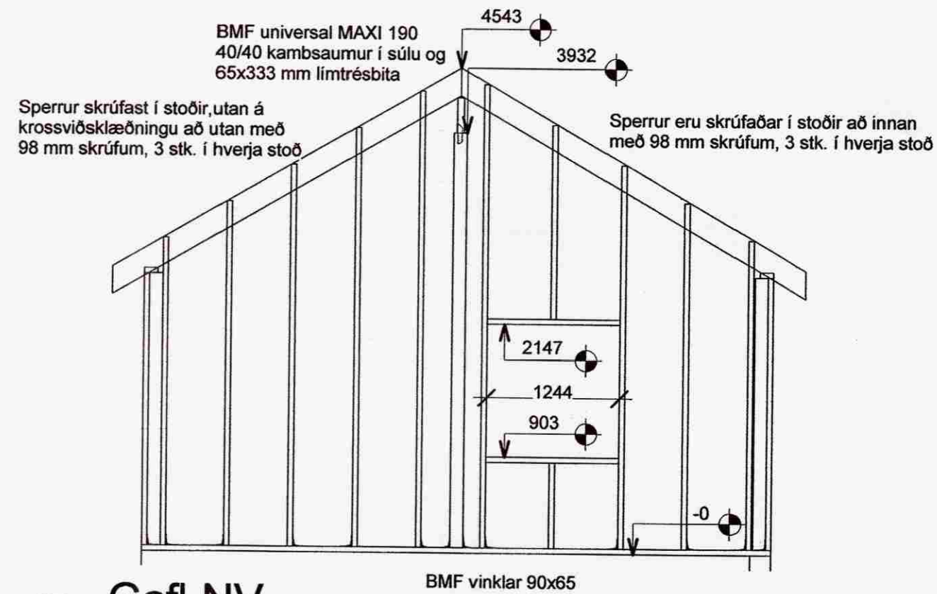
1 Gafl-NV 1 : 50
