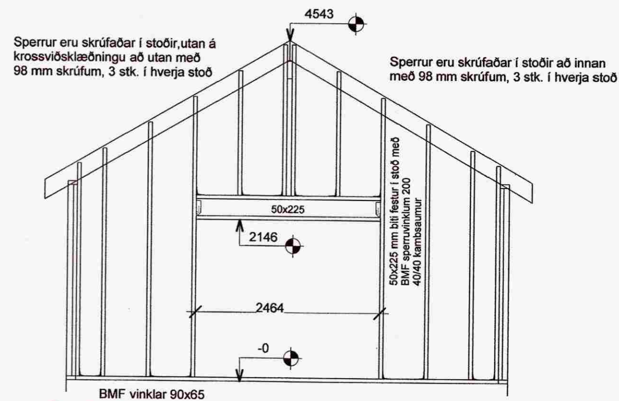
3 Gafl-SV1 1 : 50
