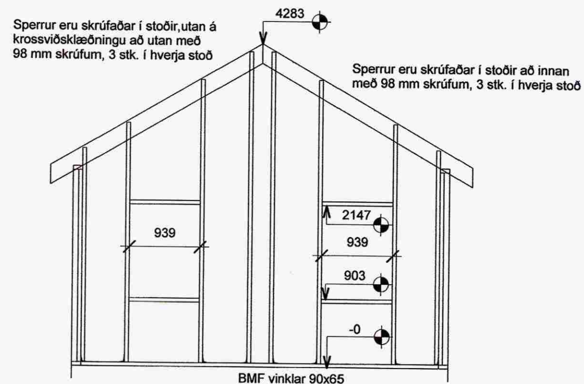
4 Gafl-SV2 1 : 50
