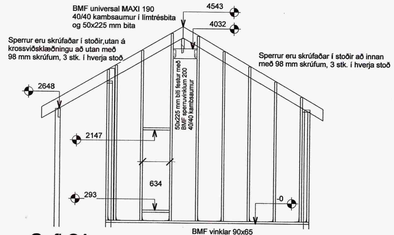
2 Gafl-SA 1 : 50
