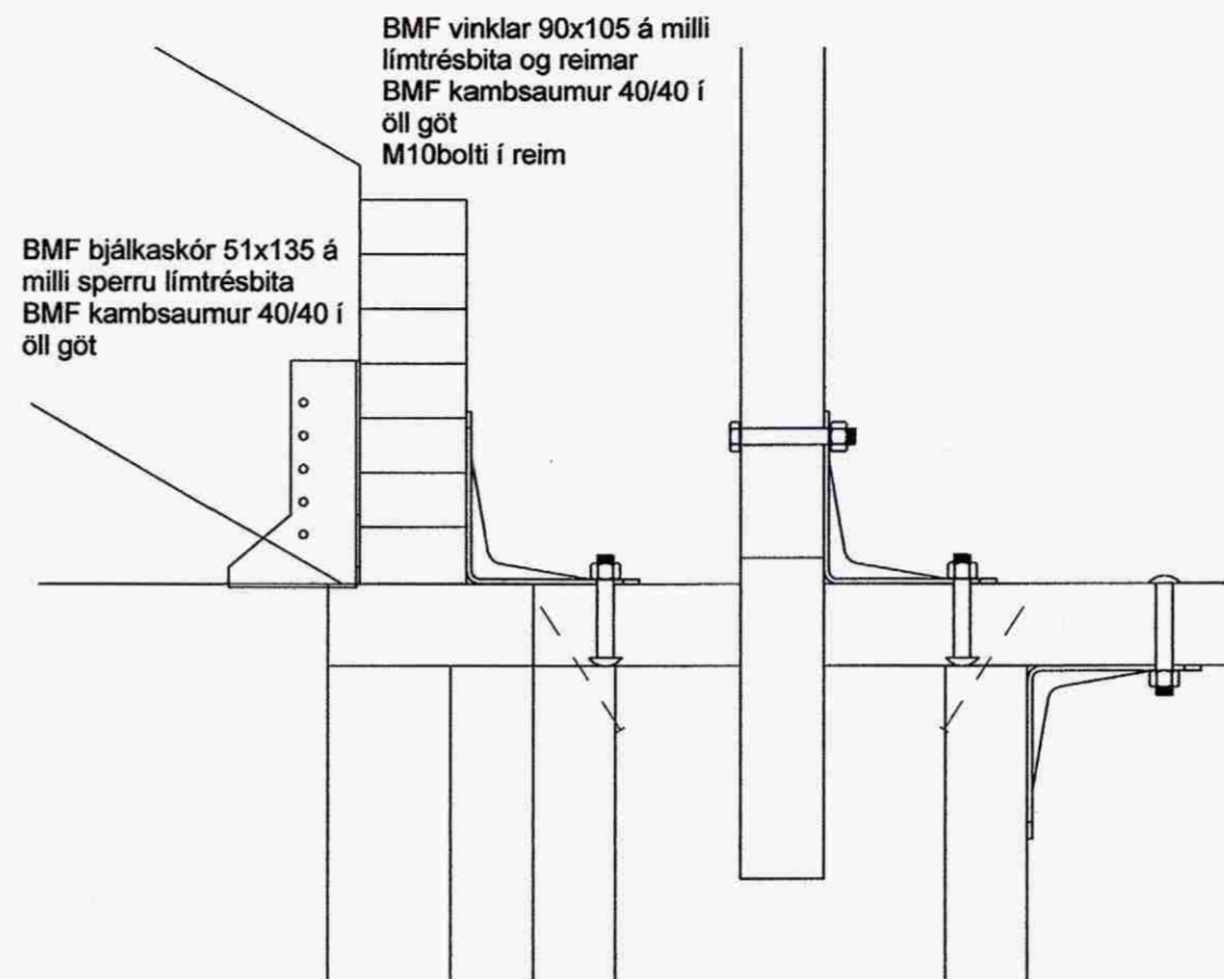
3 B-27.05.03 1:5
