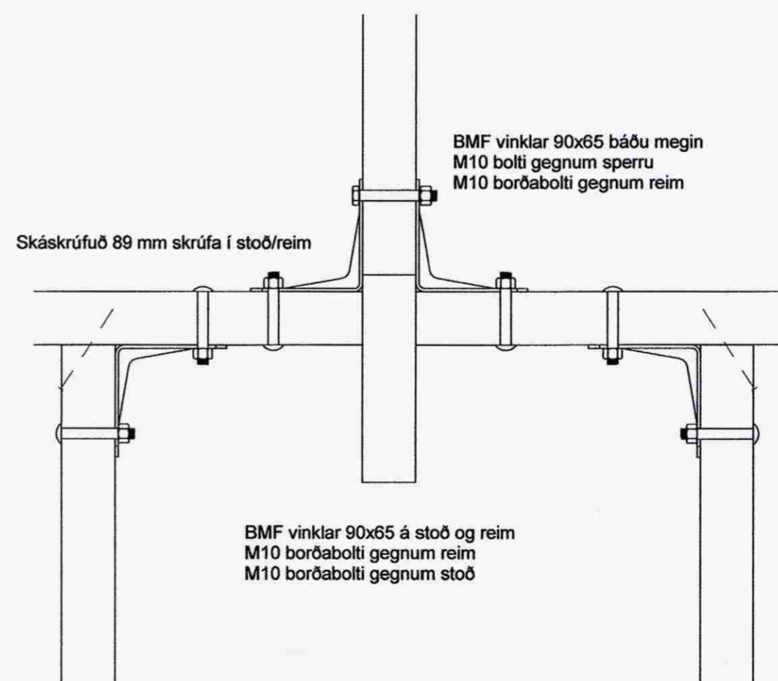
2 B-27.05.02 1:5
