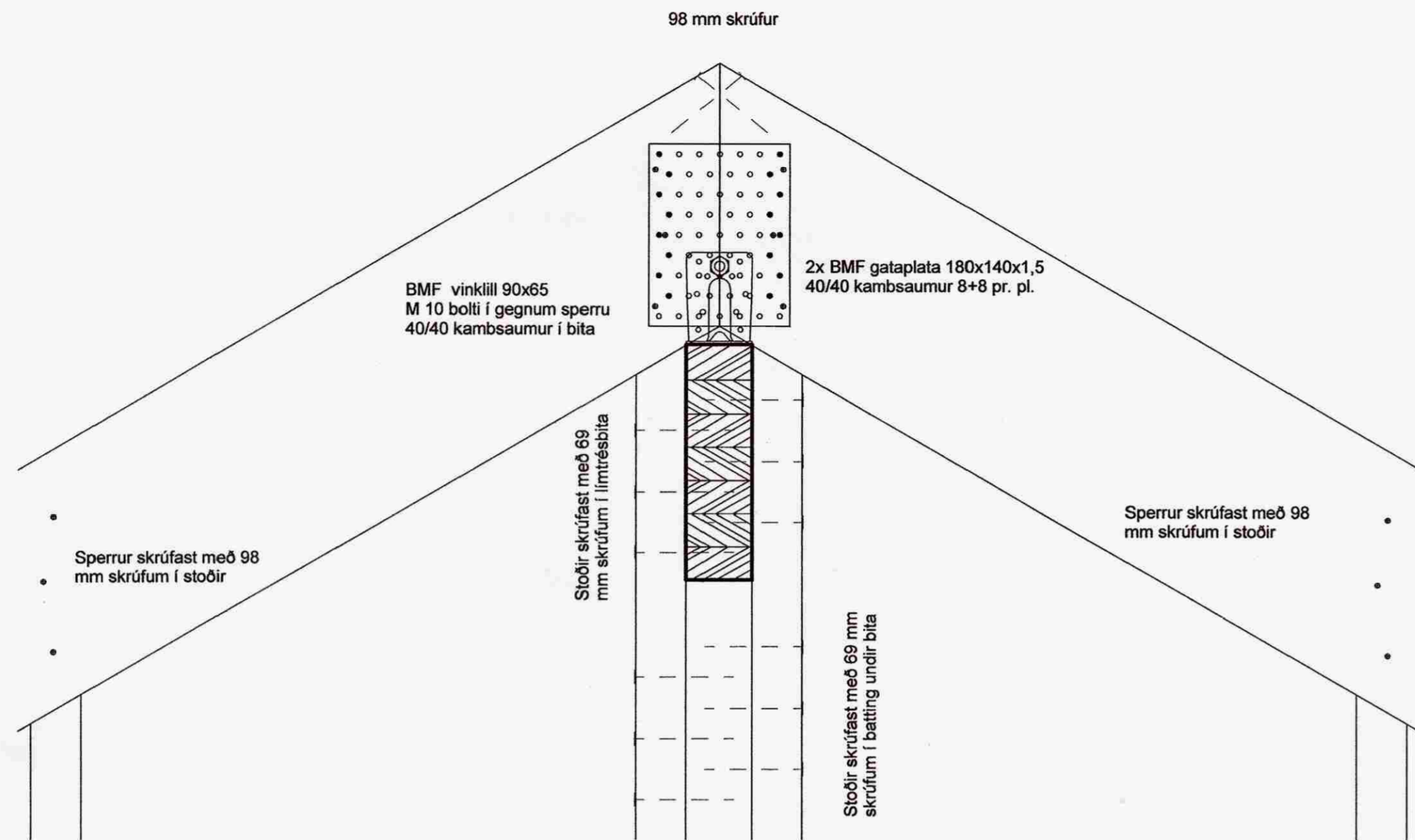
4 B-27.05.04 1:5
