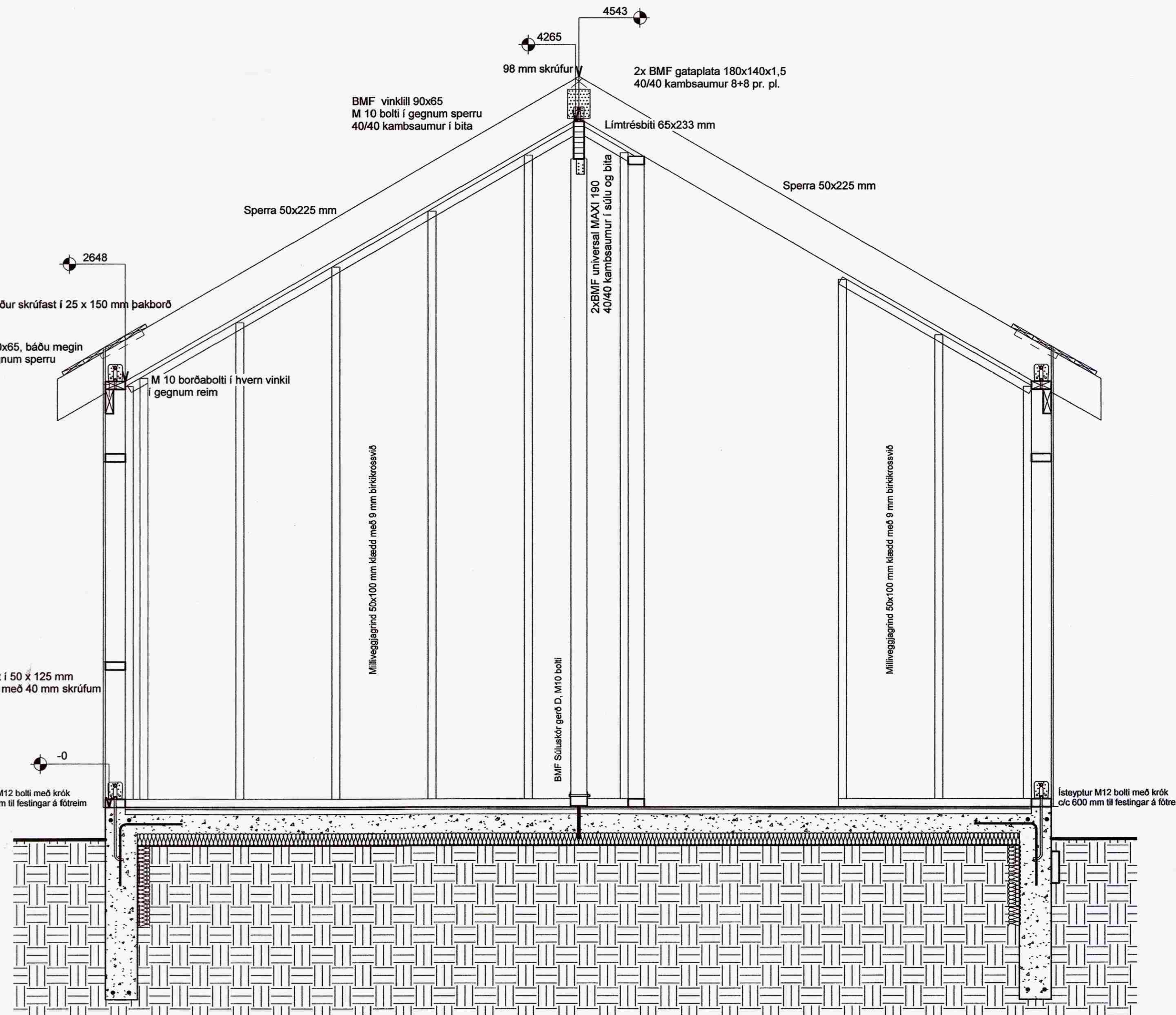
1 Skurður A 1 : 20
