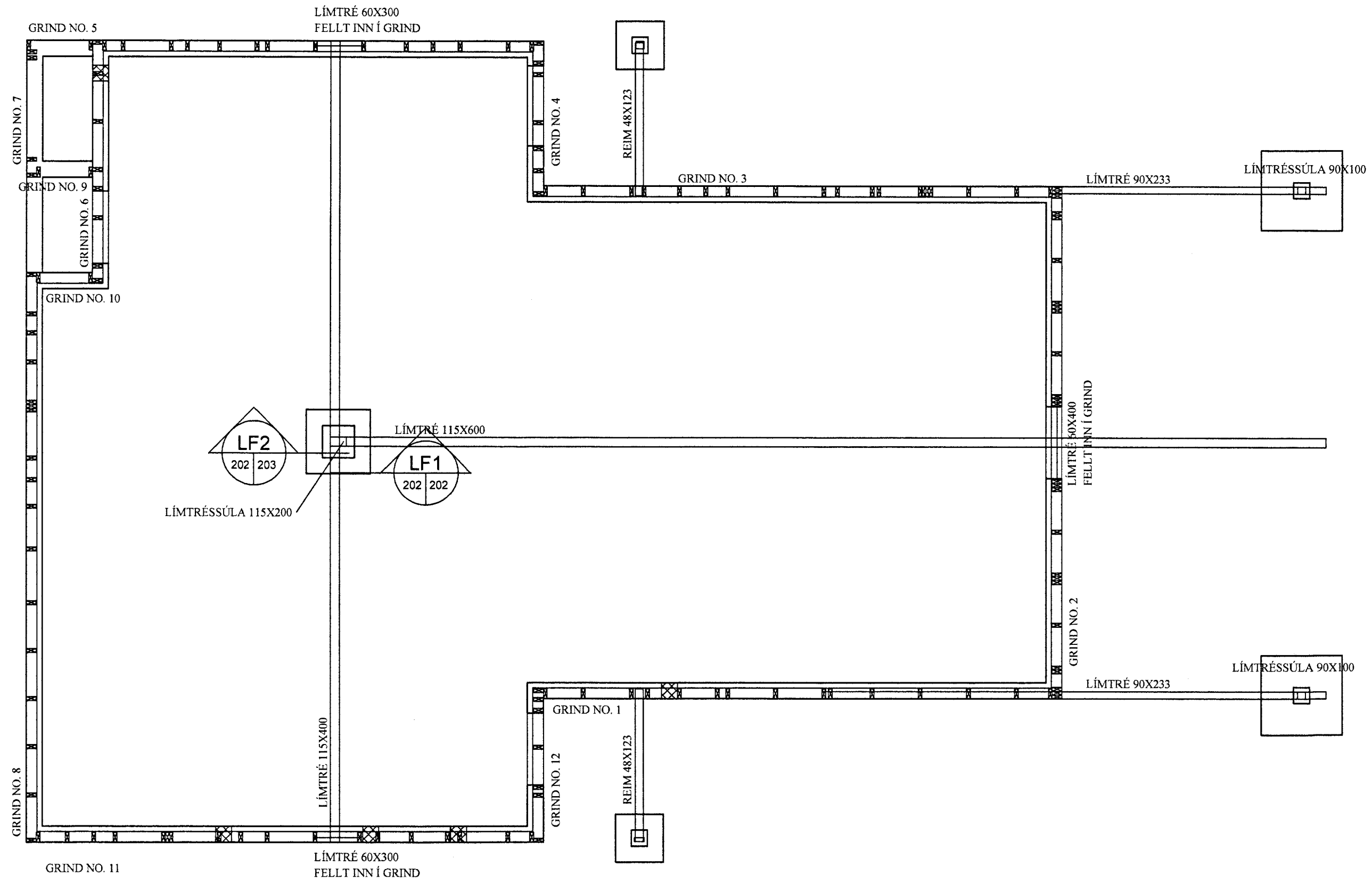
GRUNNMYND LIMTRÉ
