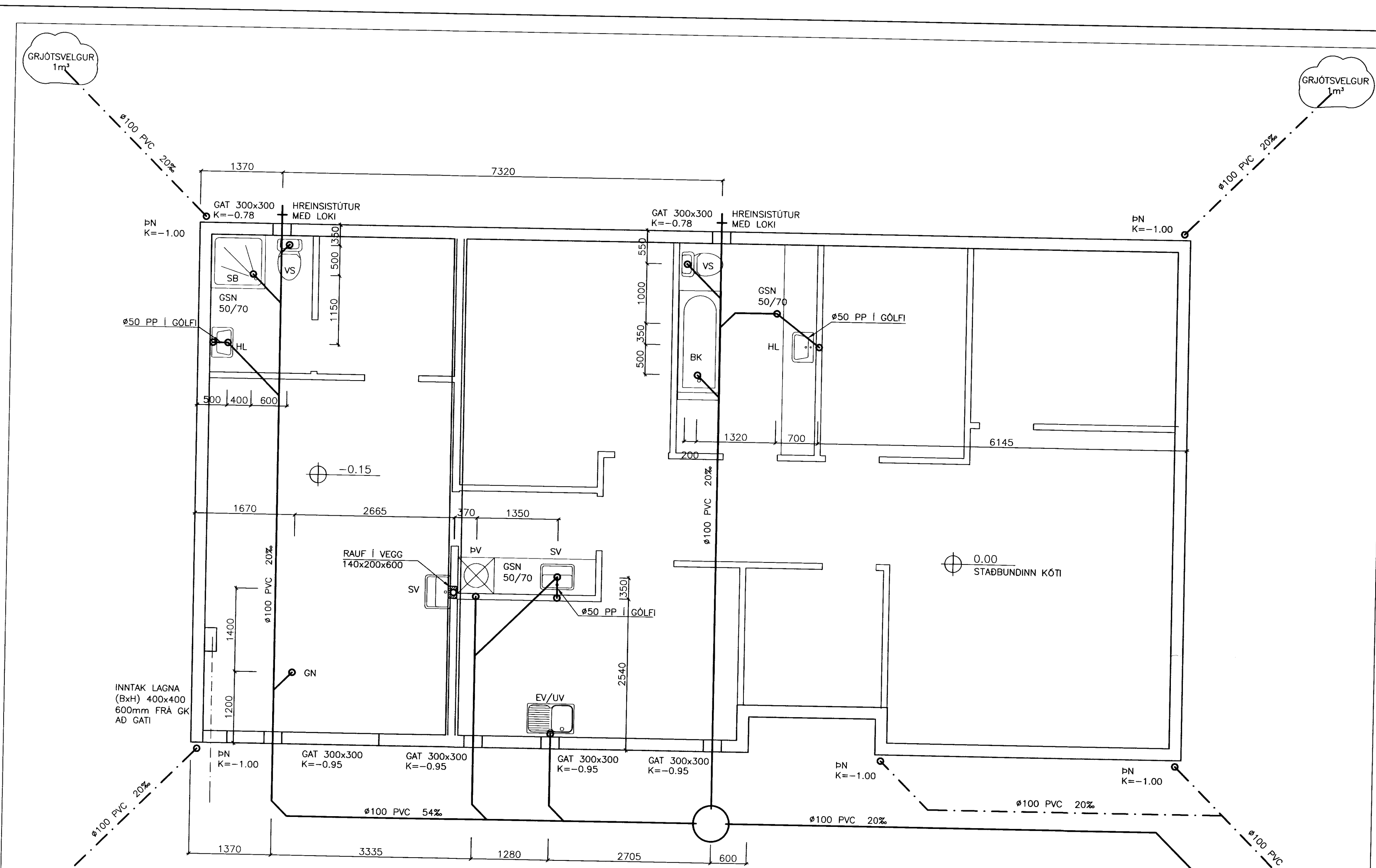
GRUNNMYND FRÁRENNISLAGNA Mkv. 1:50
