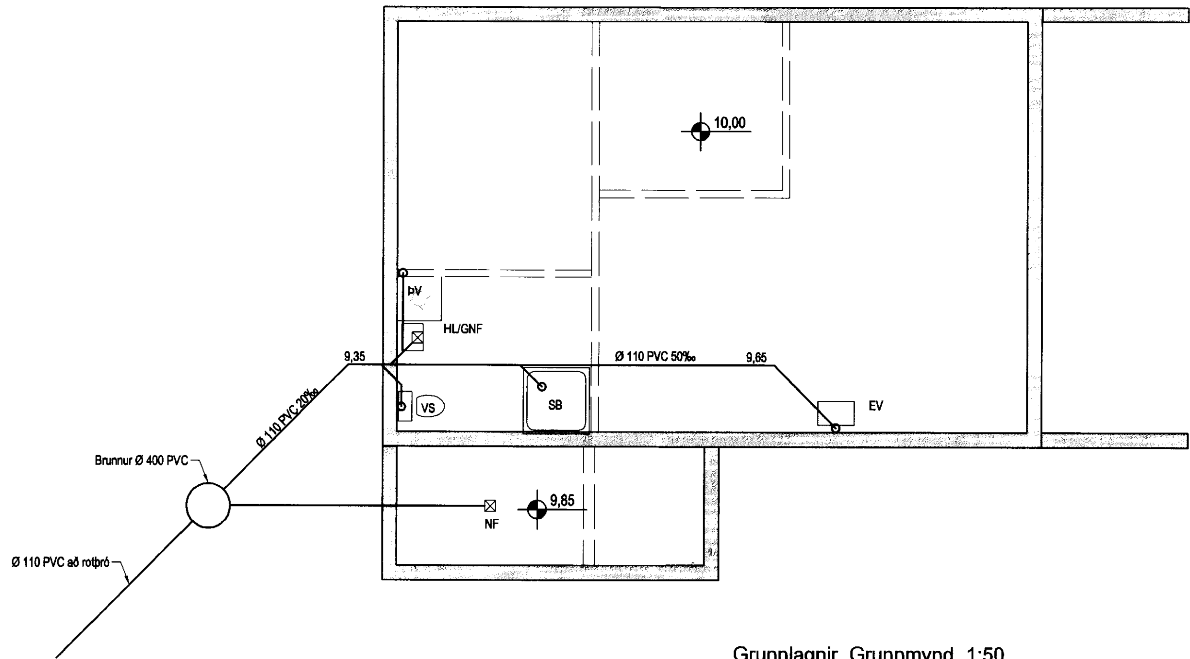
Grunnlagnir, Grunnmynd, 1:50
