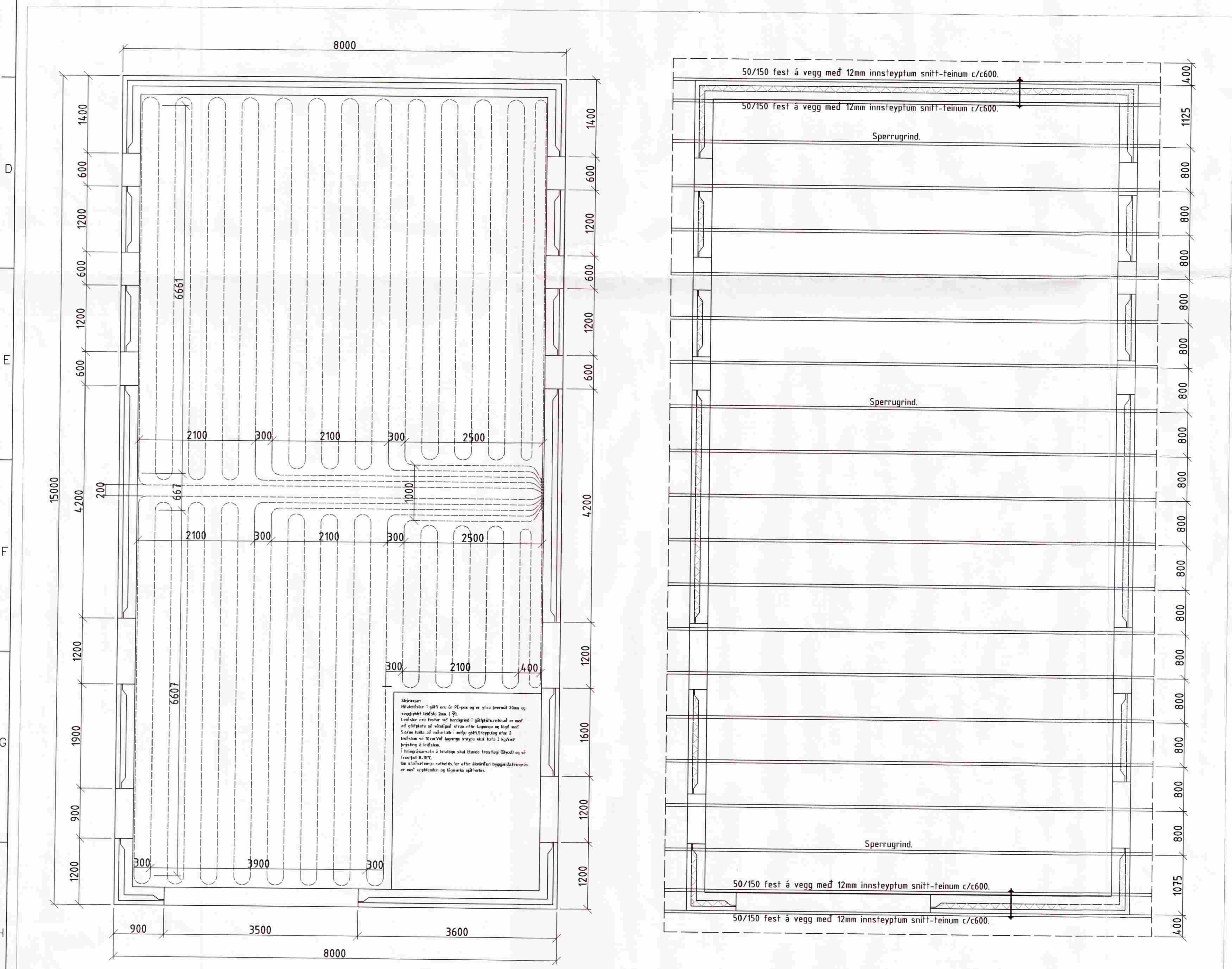
Grunnmynd-hitun
