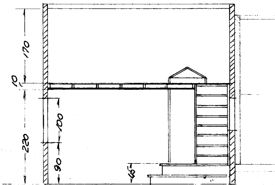
Snid A-A
