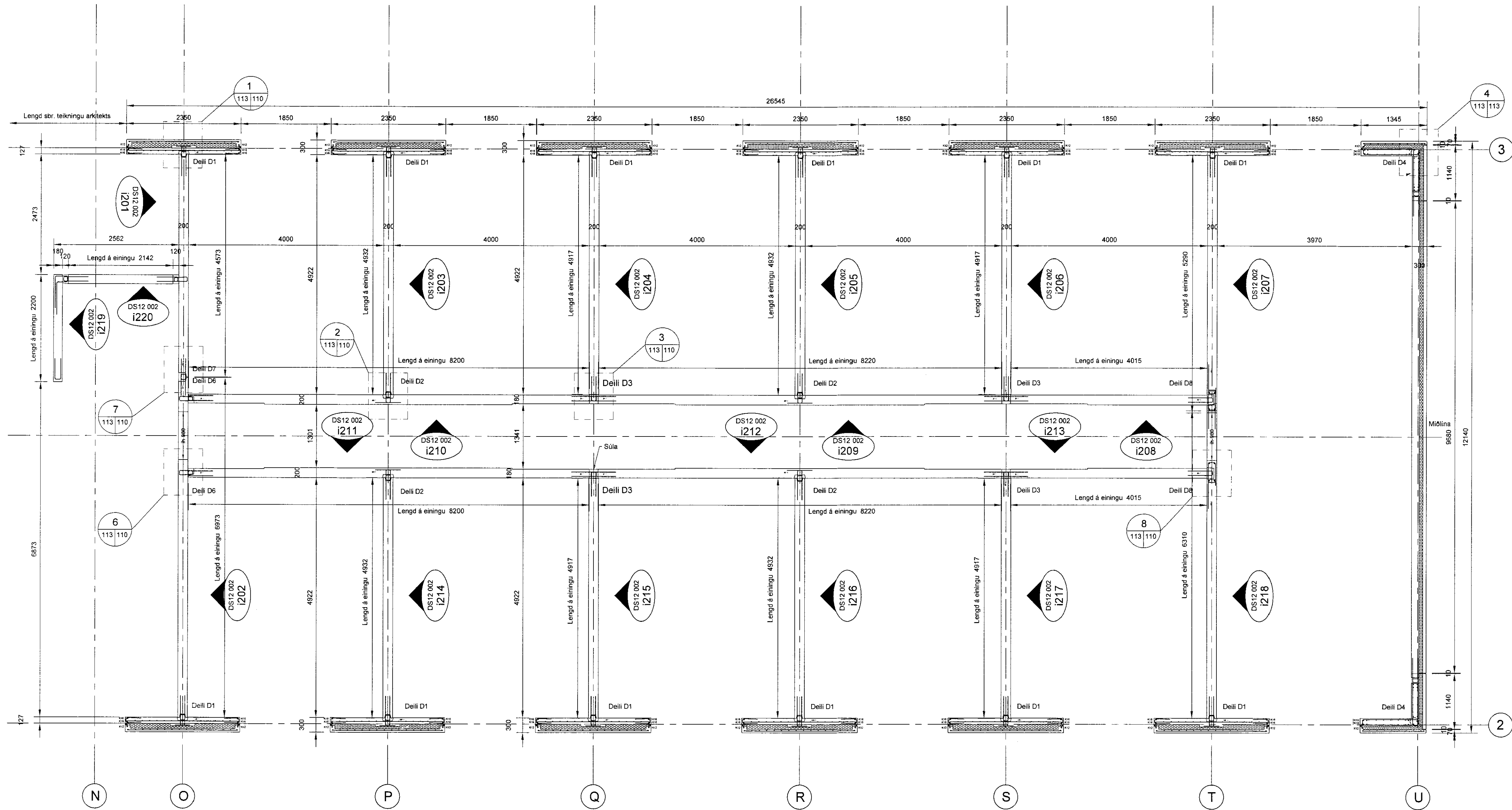
Grunnmynd 1:50
