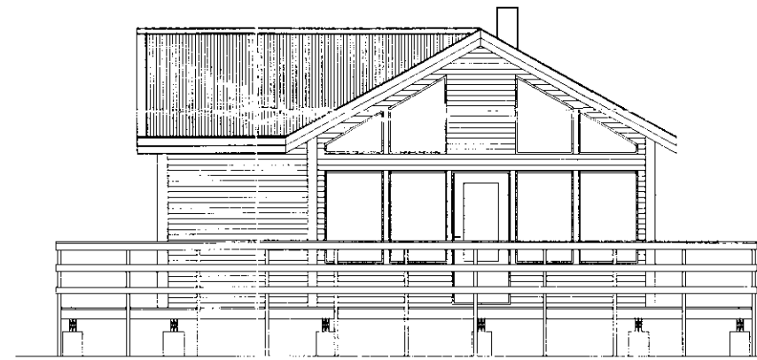
NORÐAUSTUR 1:100
