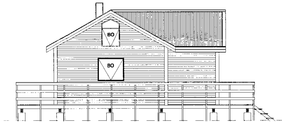
SUÐVESTUR 1:100
