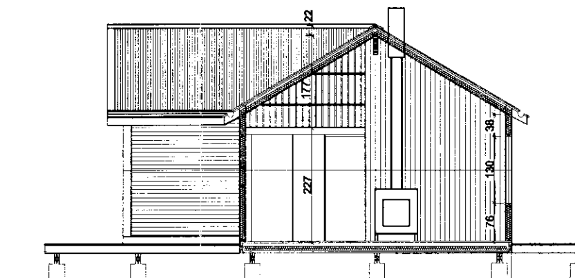
SNEIÐING A-A 1:100
