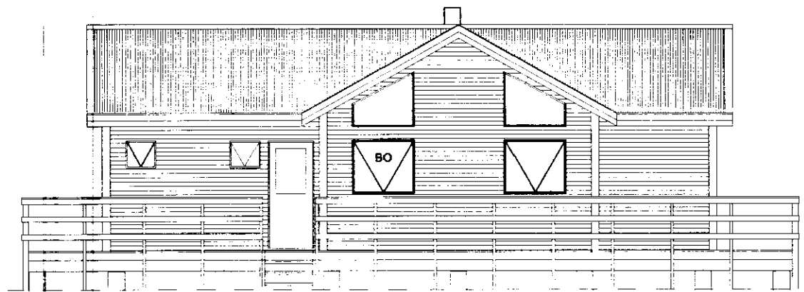
SUÐAUSTUR 1:100
