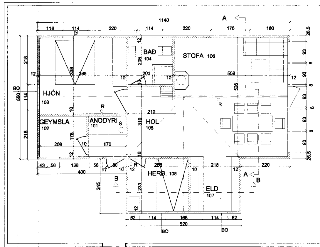
GRUNNMYND 1:100
