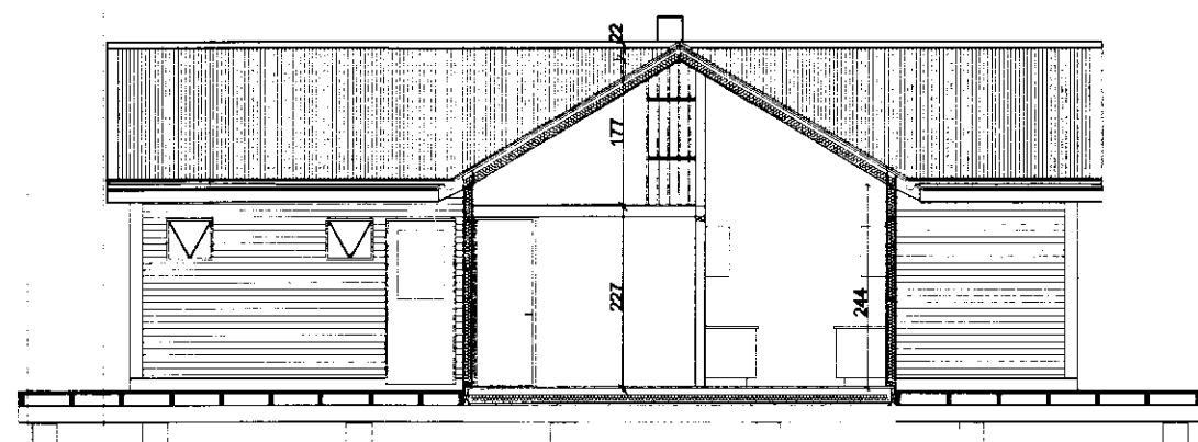
SNEIÐING B-B 1:100
