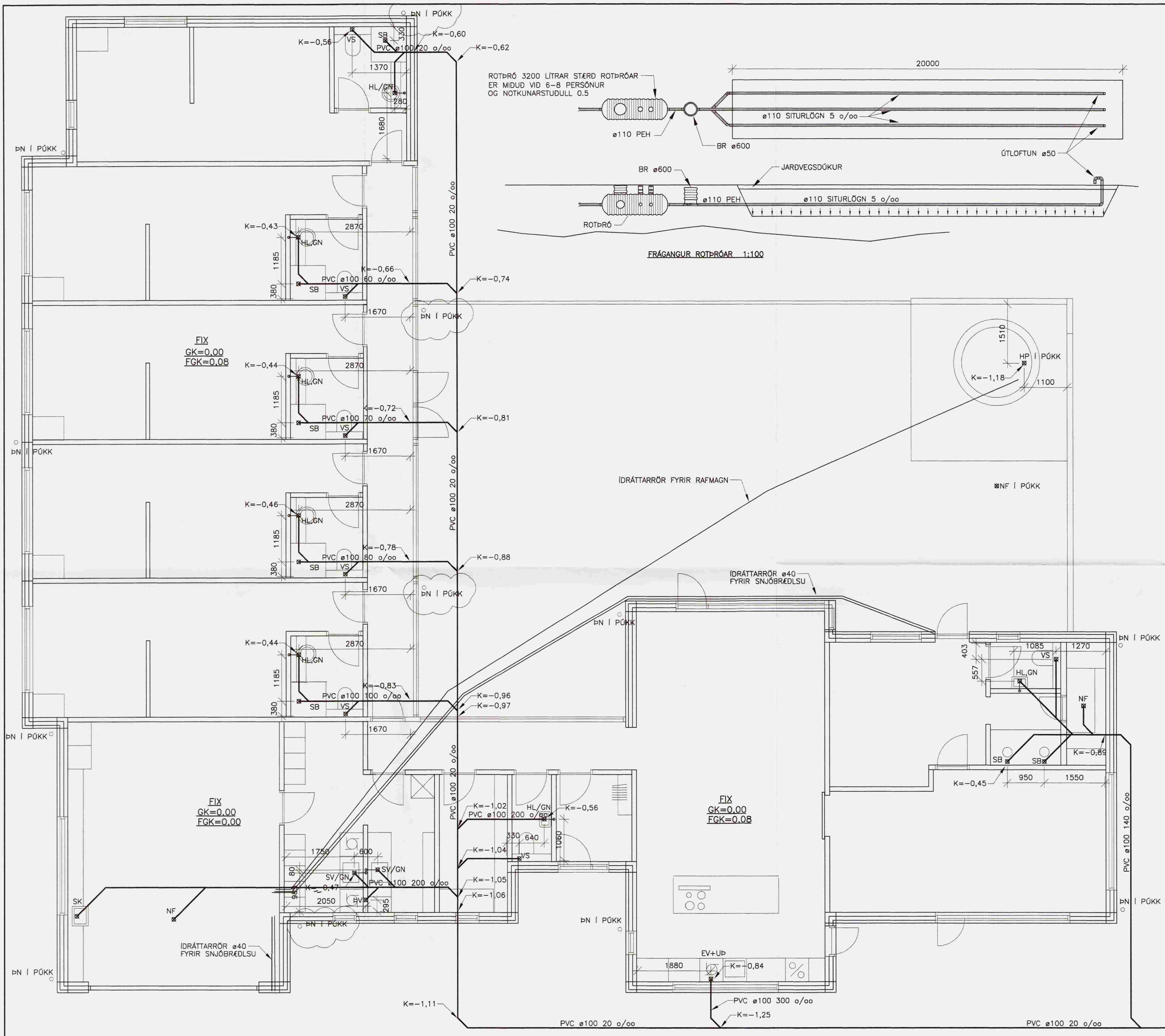
GRUNNMYND, 1:50
