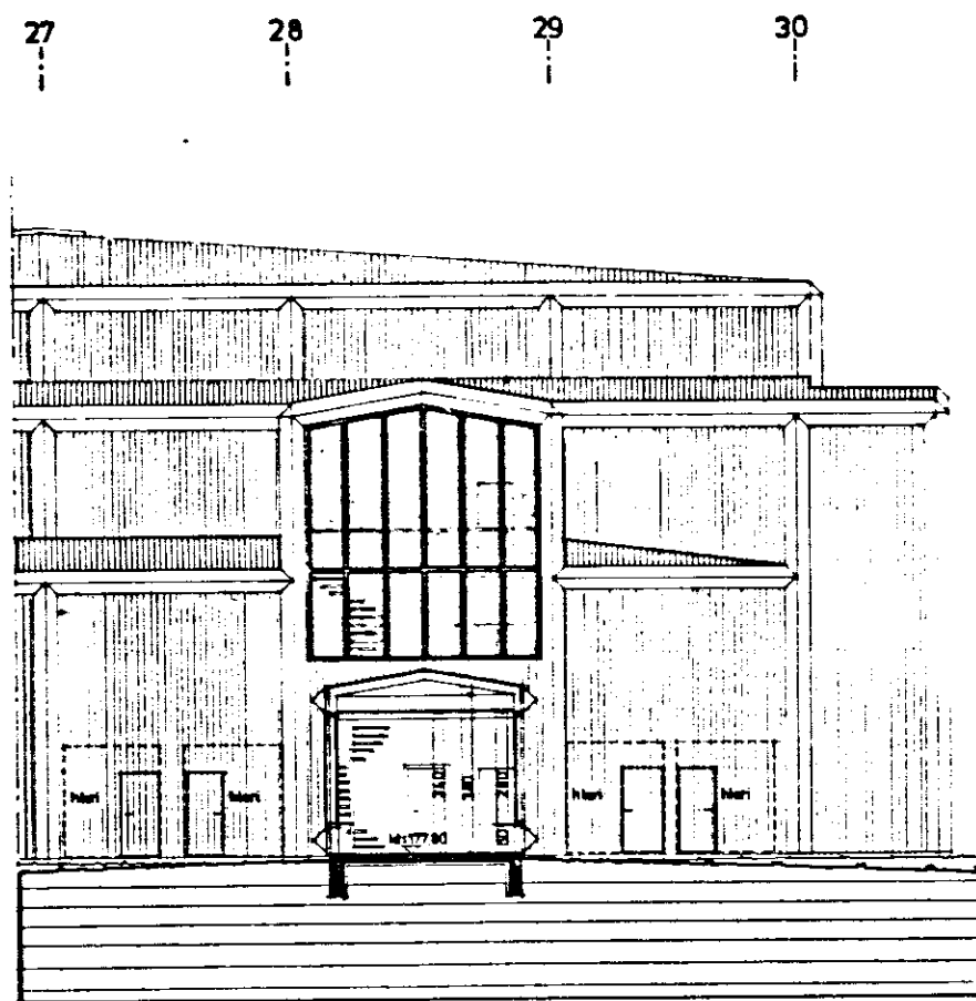
sneiding E-E
