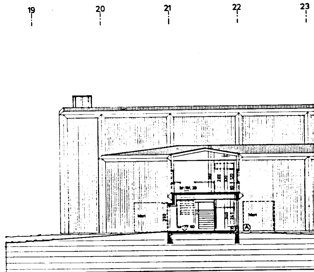
sneiding D-D
