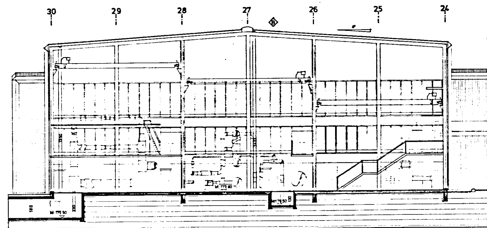
sneiding G-G
