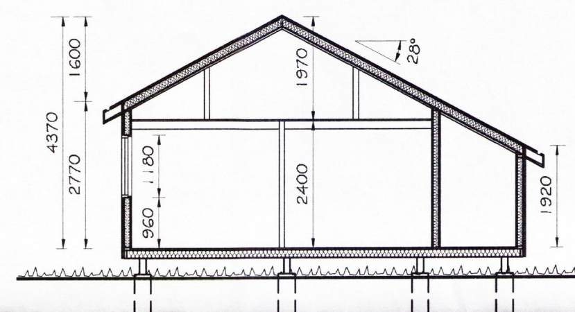
SNÍÐ B-B mkv. 1:100
