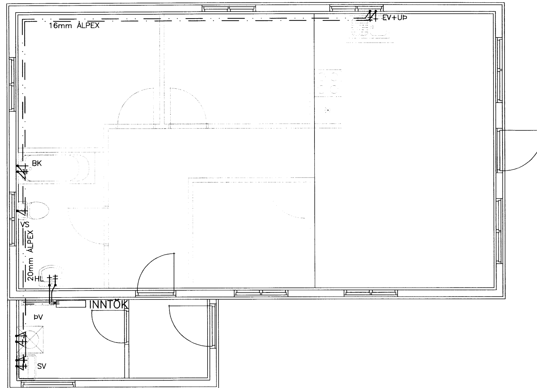
NEYSLUVATNSLAGNIR GRUNNMYND MKV. 1:50
