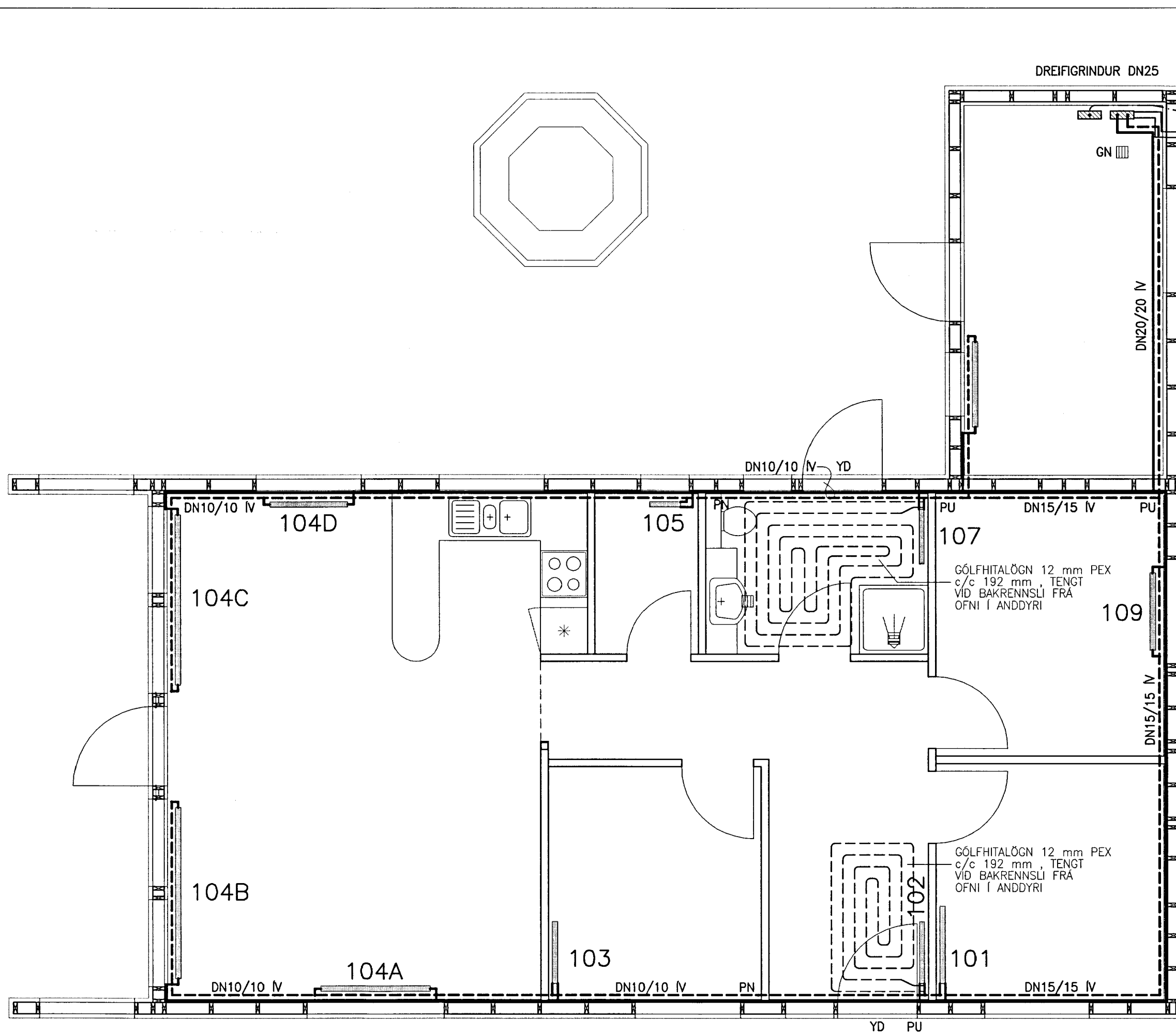
GRUNNMYND HITALAGNIR 1:50
