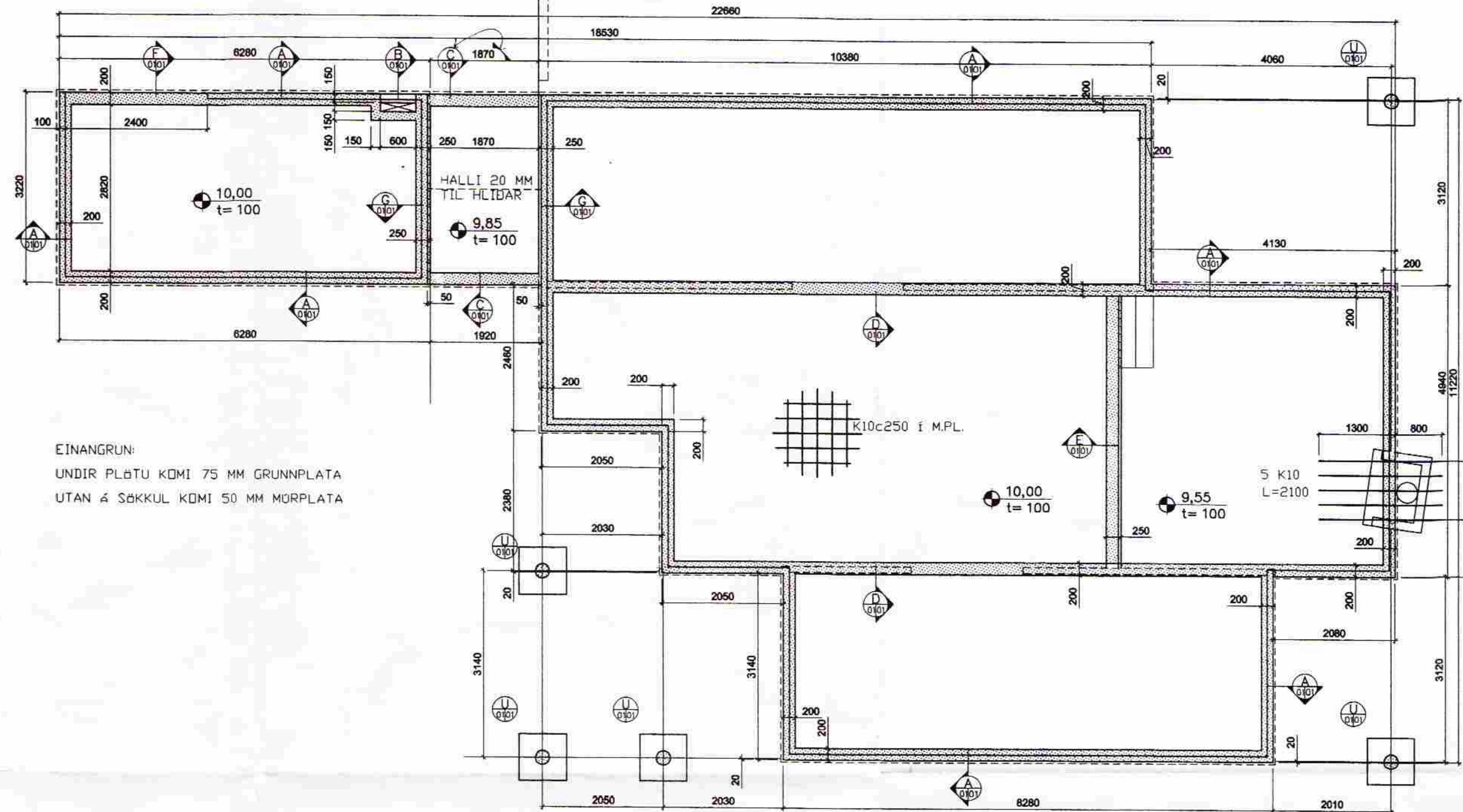
SÖKKLAR, GRUNNMYND, 1:50
