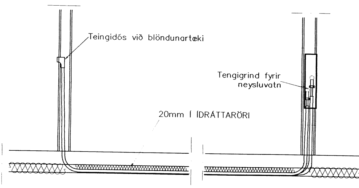
TENING NEYSLUVATNSLAGNA 1:20
