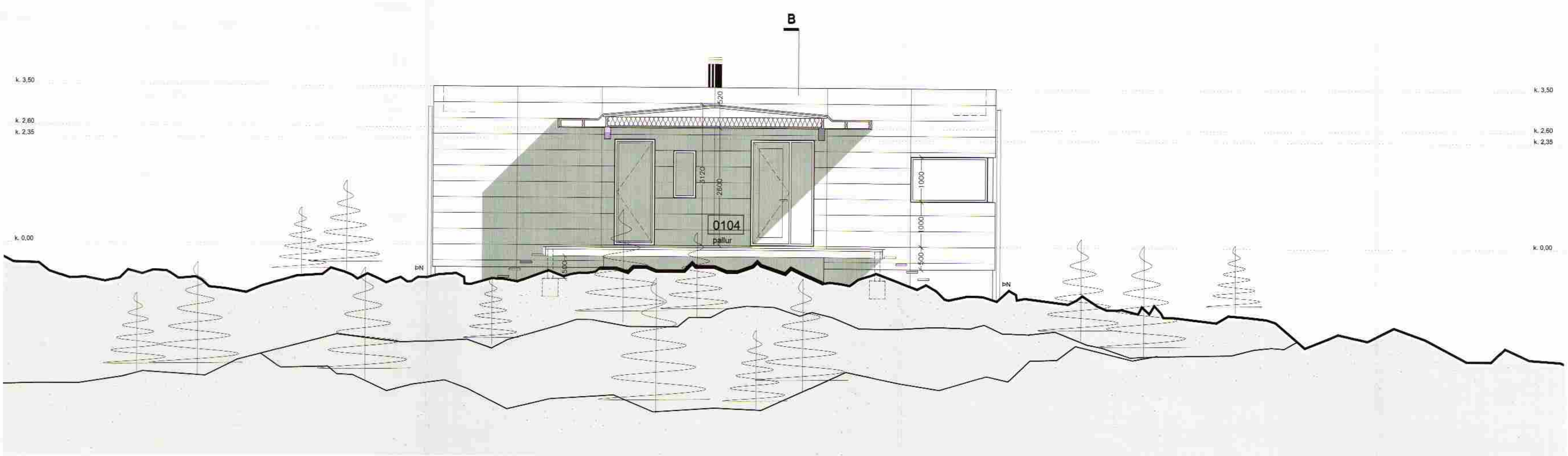
SNEIÐING D - D M 1:50
