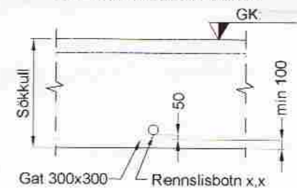
Skýringamynd af sökkulgötum
