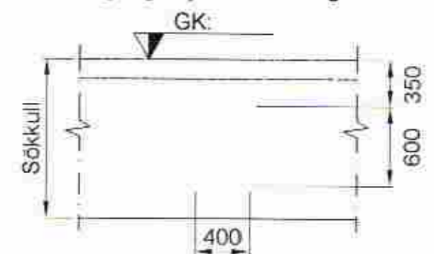
Skýringamynd af inntaksgati
