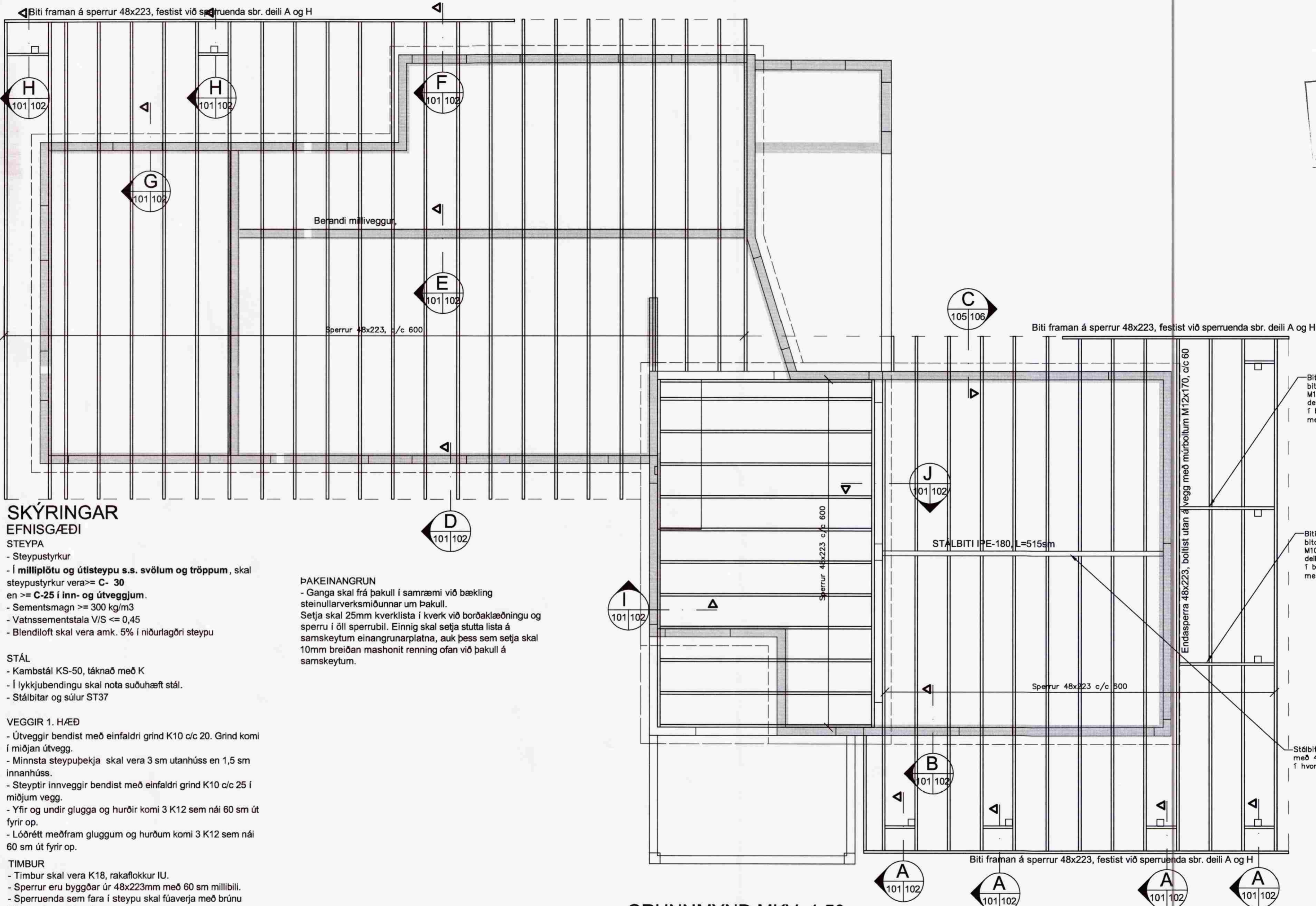
GRUNNMYND MKV. 1:50
