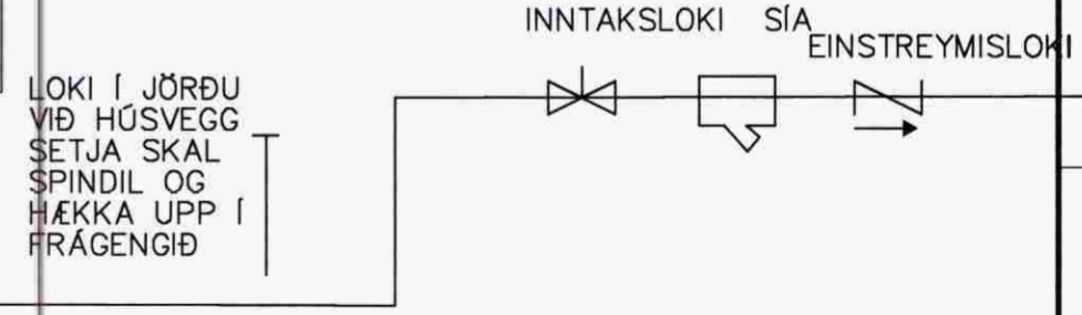
VATNSINNTAK (Skematísk mynd)
