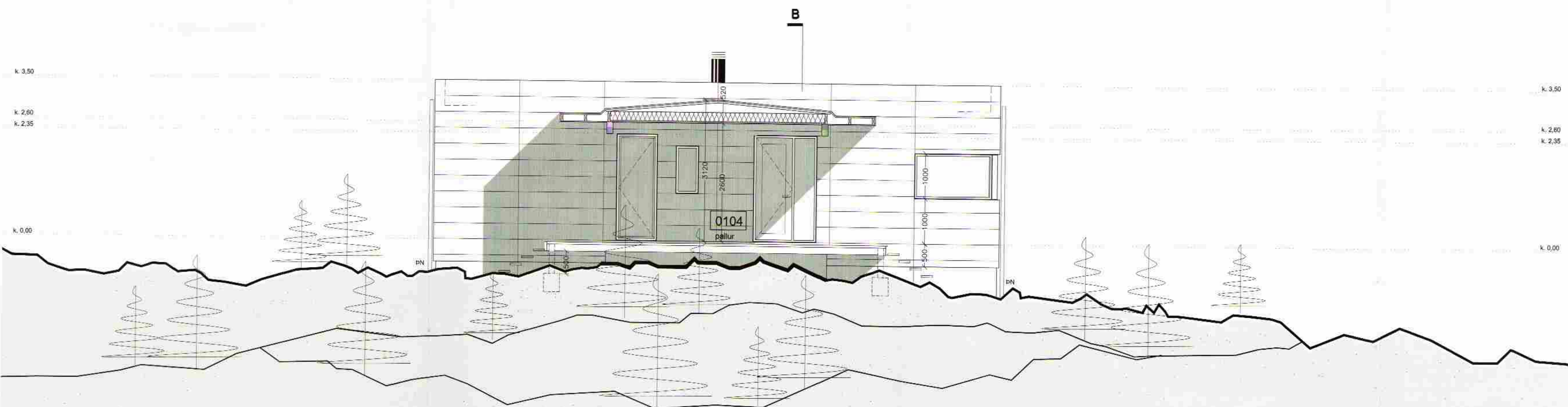
SNEIÐING D - D M 1:50
