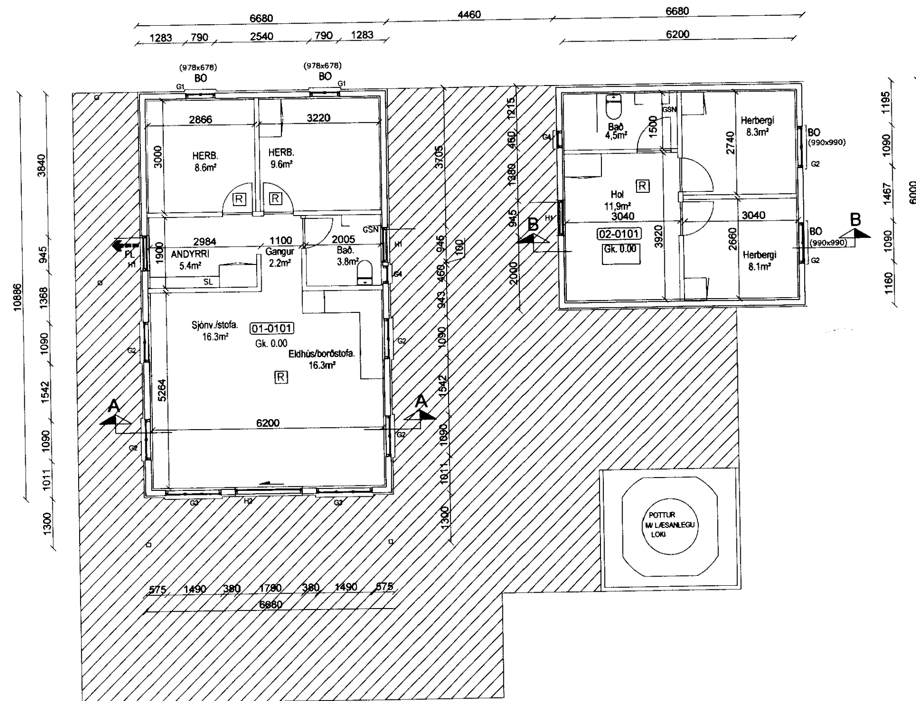
Grunnmynd Mkv. 1:100
