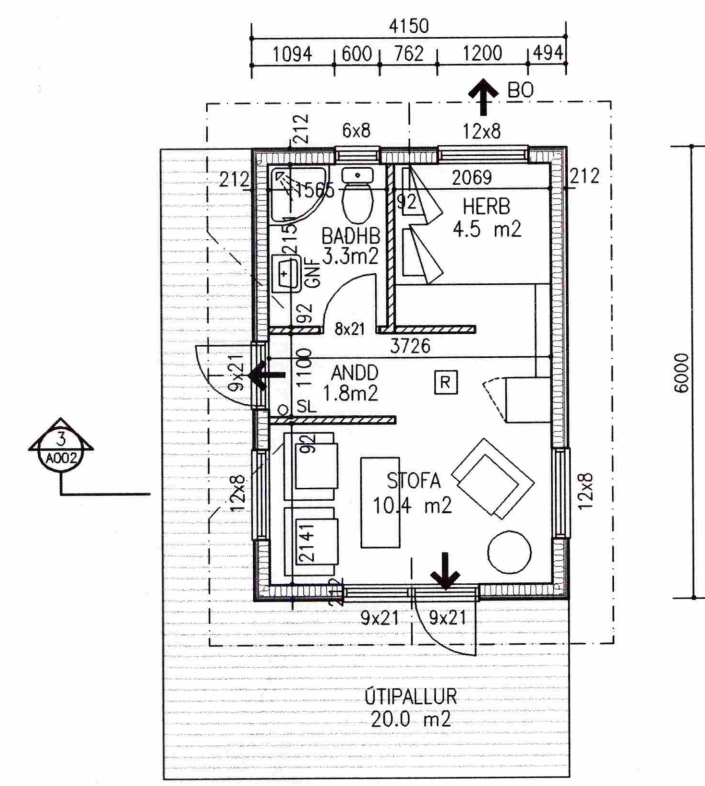
GESTAHÚS GRUNNM 1:100
