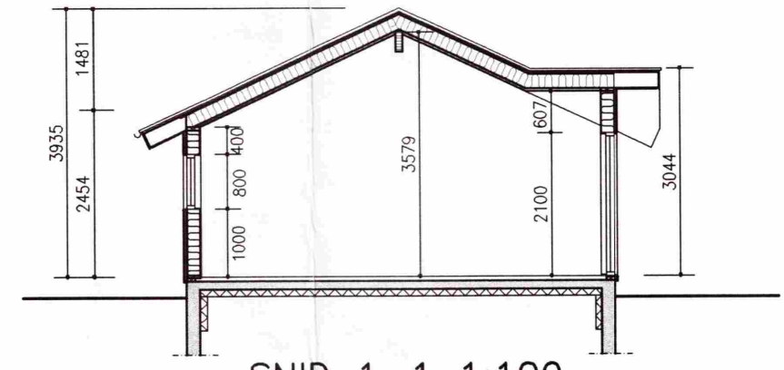
SNID 1-1 1:100
