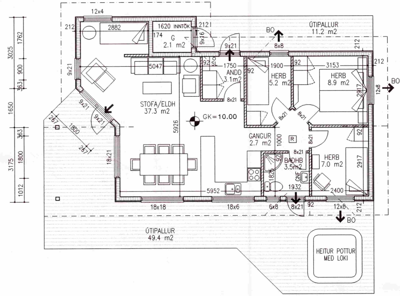
SUMARHÚS GRUNNM 1:100
