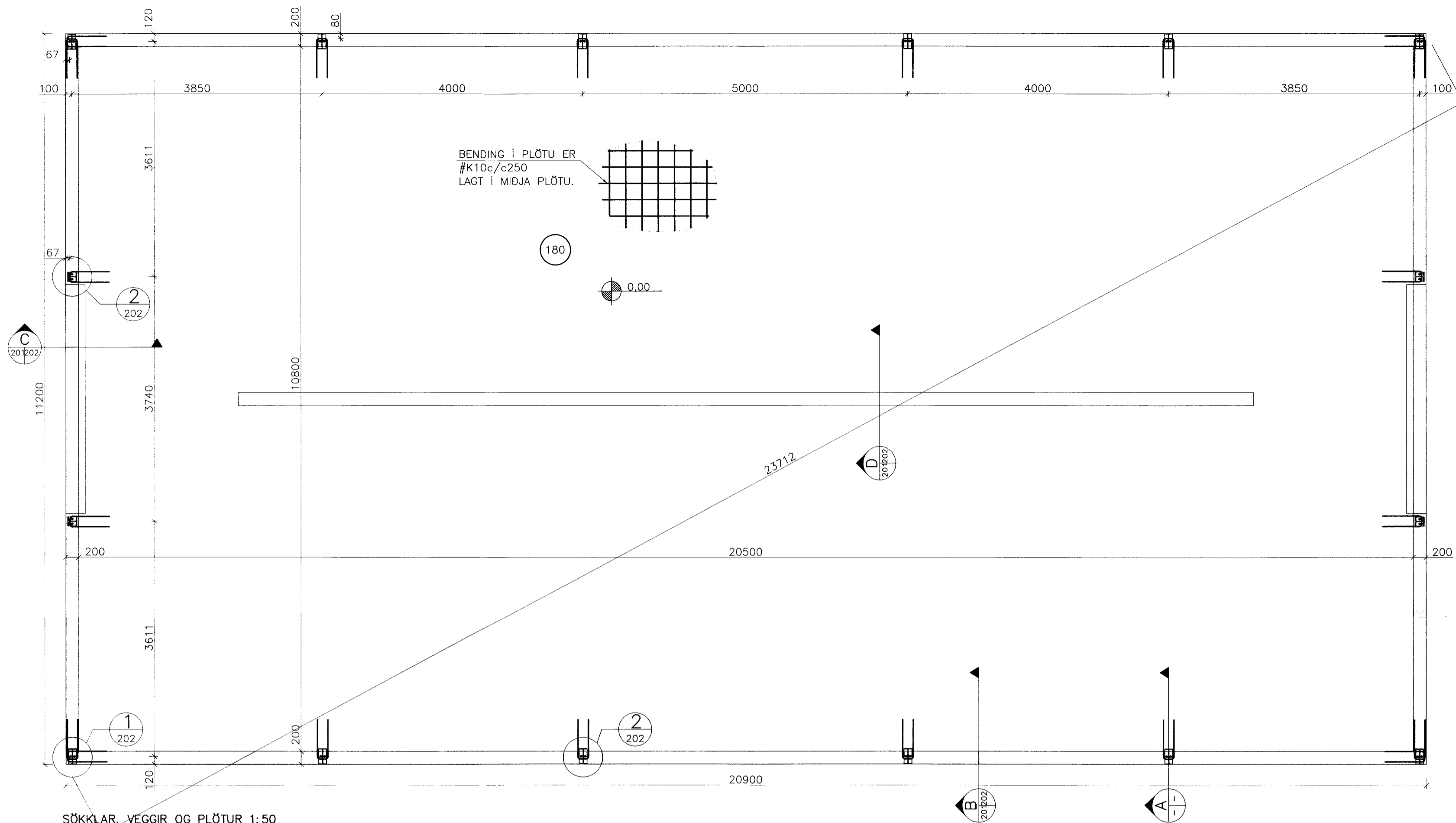
SÖKKLAR, VEGGIR OG PLÖTUR 1:50
