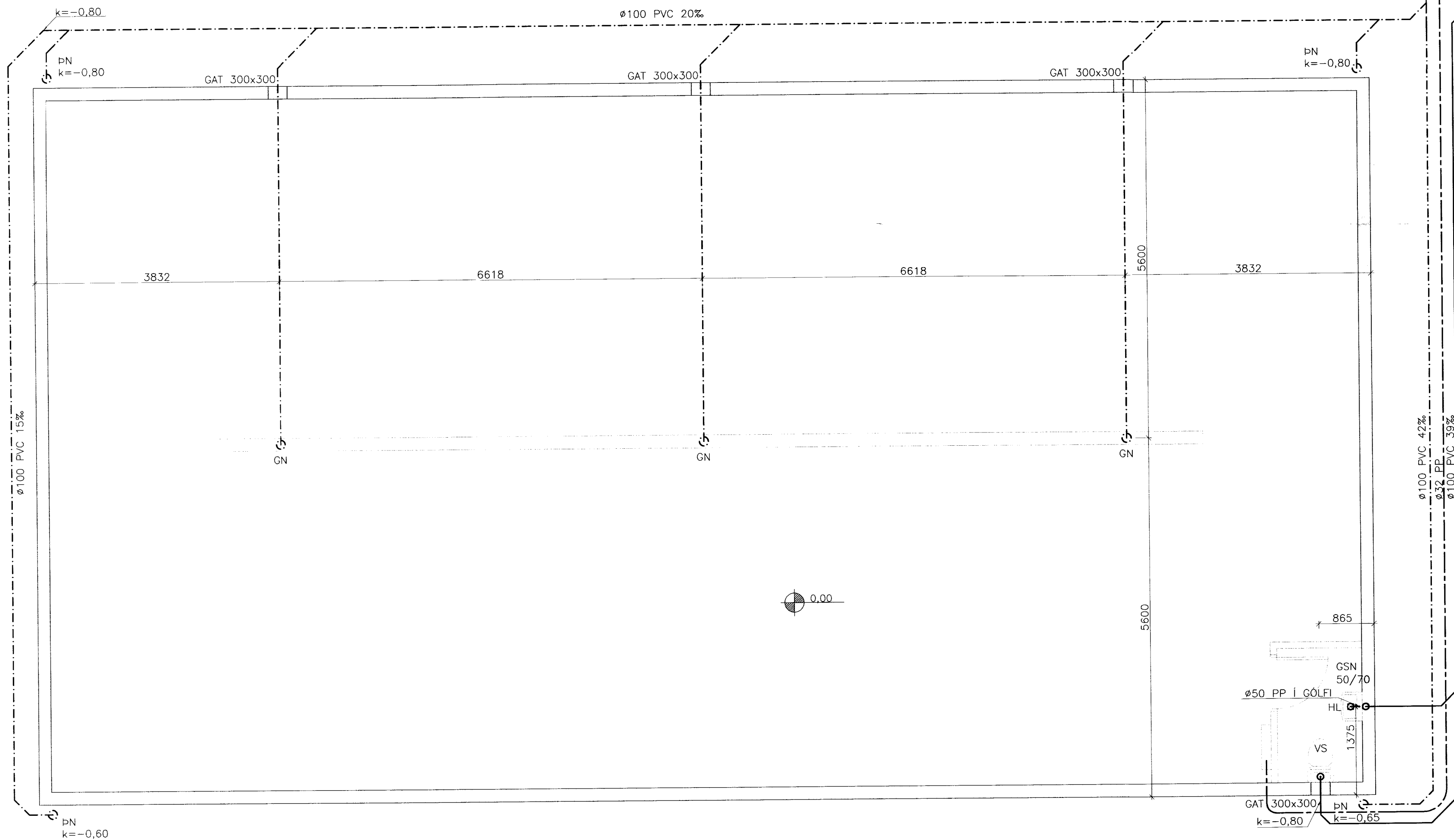
GRUNNMYND FRÆRENNSLISLAGNA 1:50
