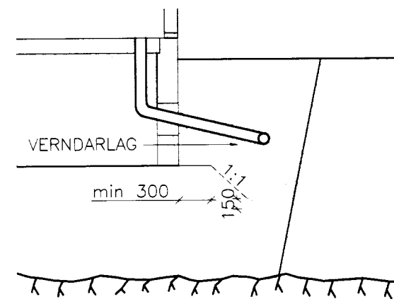
SNID VIÐ SÖKKUL 1:50
