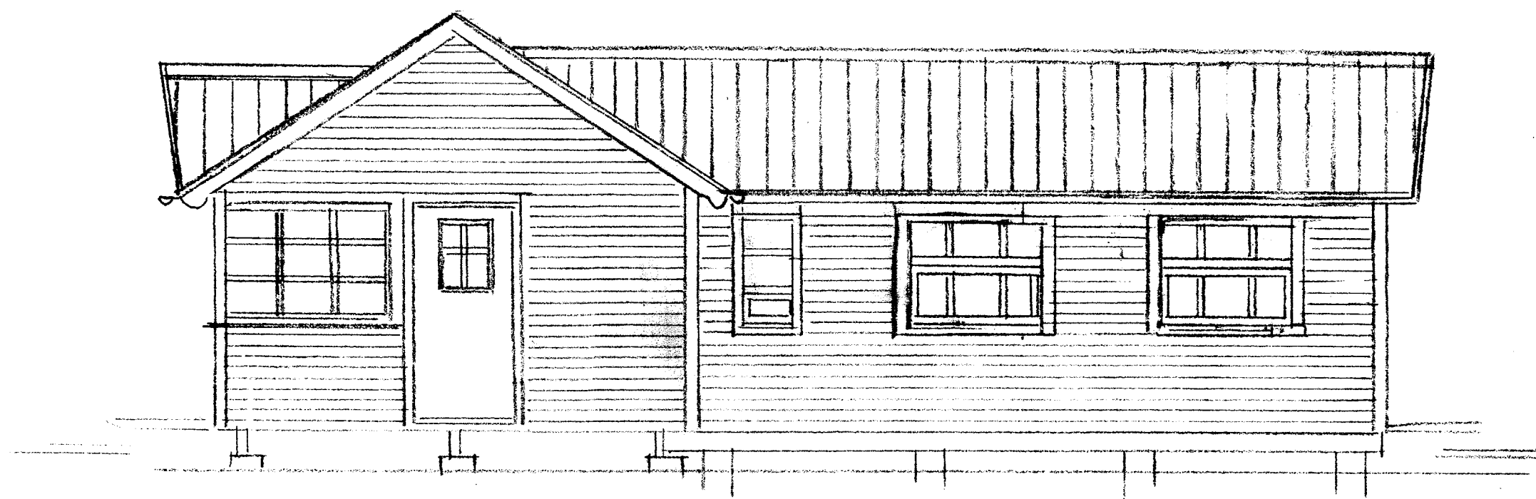
Vestur 1:50
