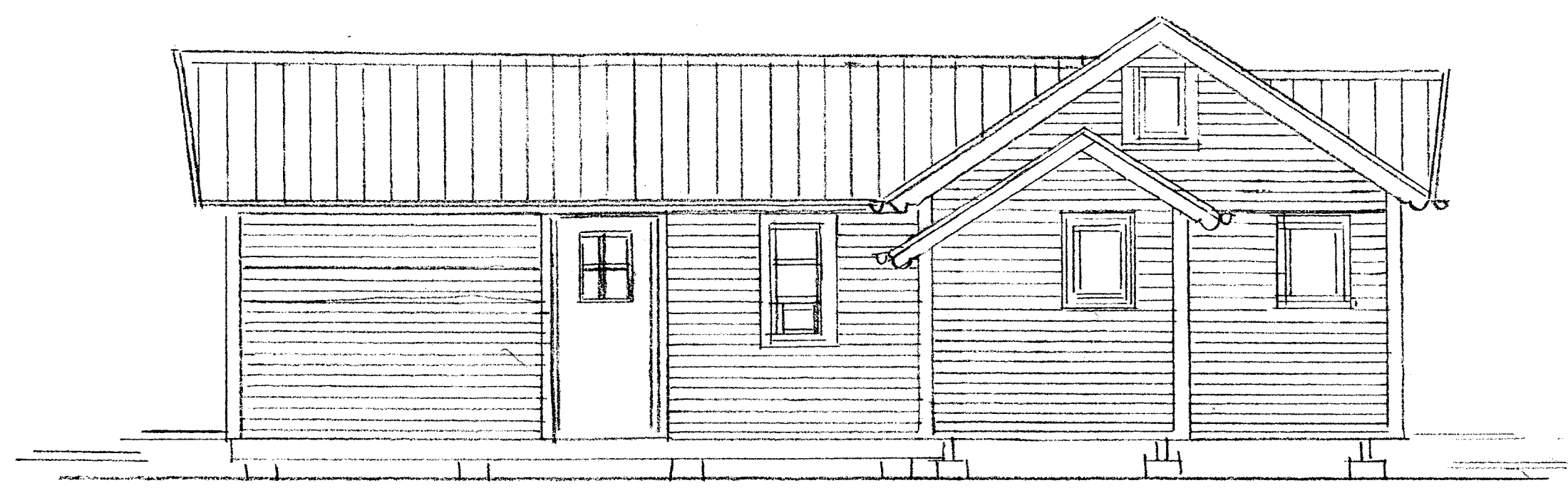
Austur 1:50
