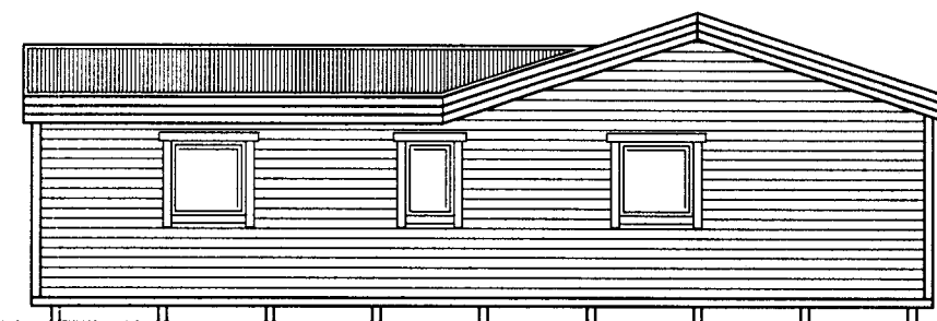
AUSTURHLID 1:100
