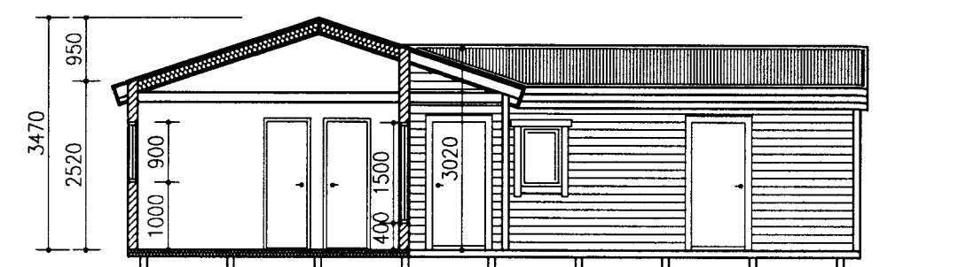
SNID 1-1 1:100
