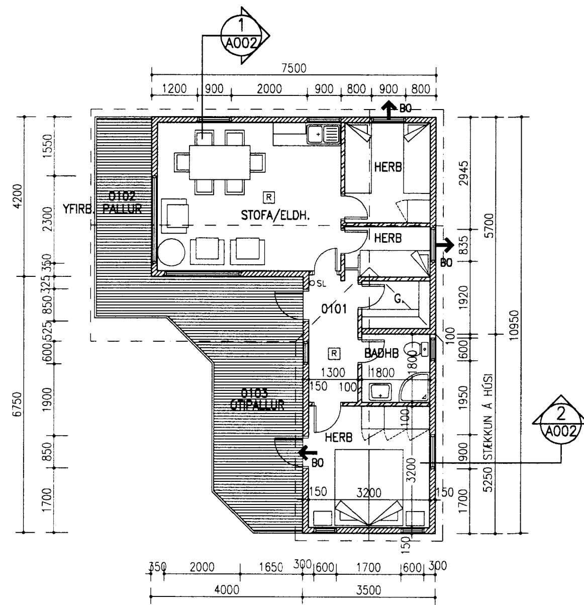
GRUNNMYND 1. HÆÐ 1:100
