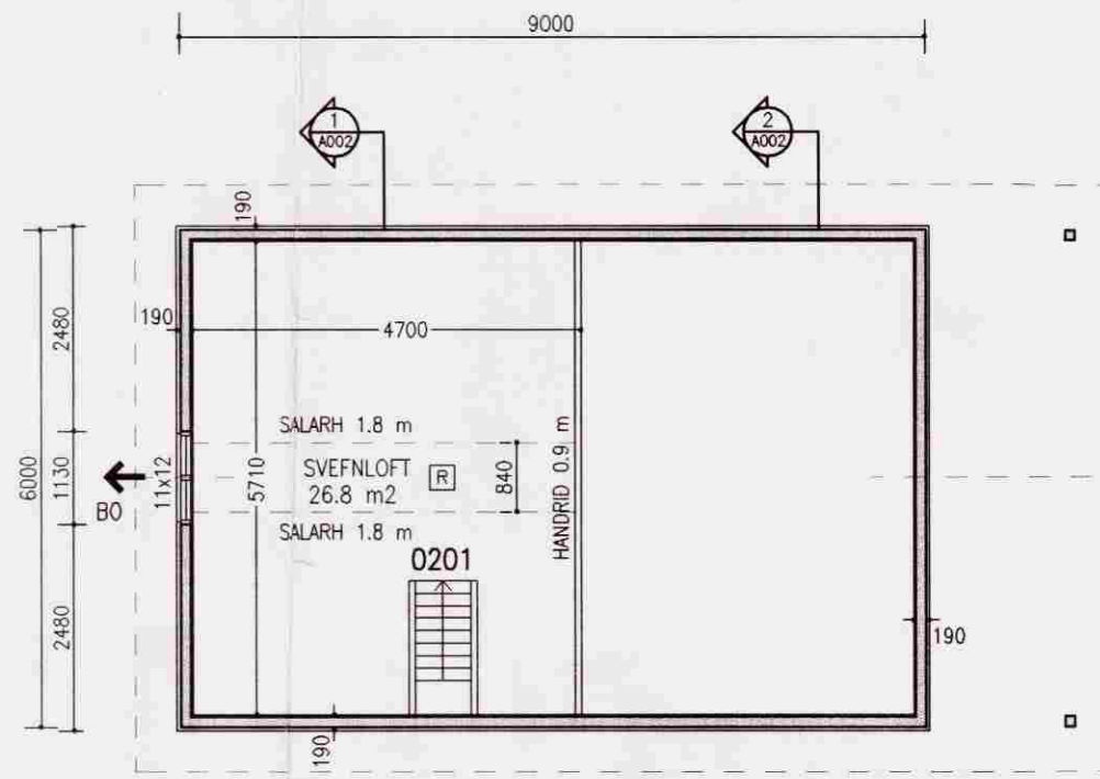
GRUNNMYND SVEFNLOFT 1:100
