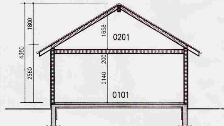
SNID 1-1 1:100
