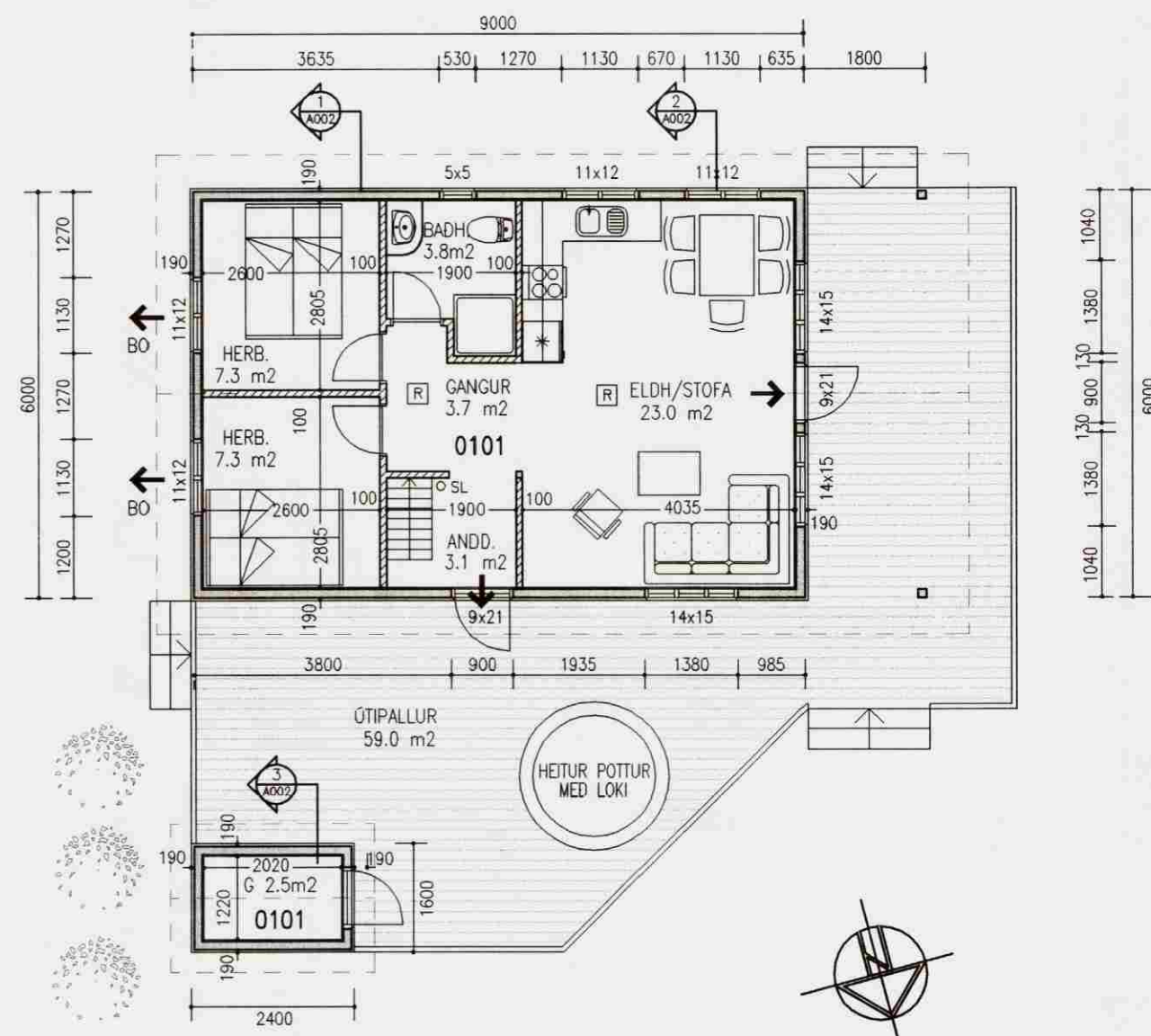
GRUNNMYND1. HÆÐ 1:100
