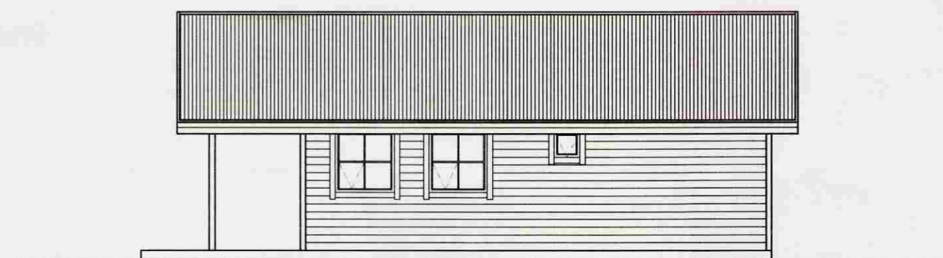
ÚTLIT SUÐURHLIÐ
