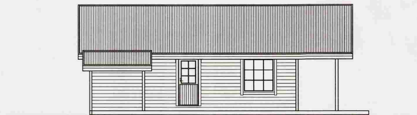
ÚTLIT NORDURHLIÐ
