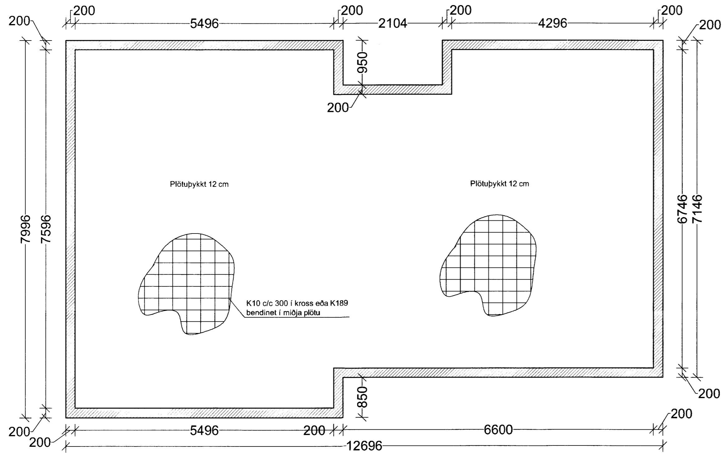
SÖKKULGRUNNMYND 1:50
