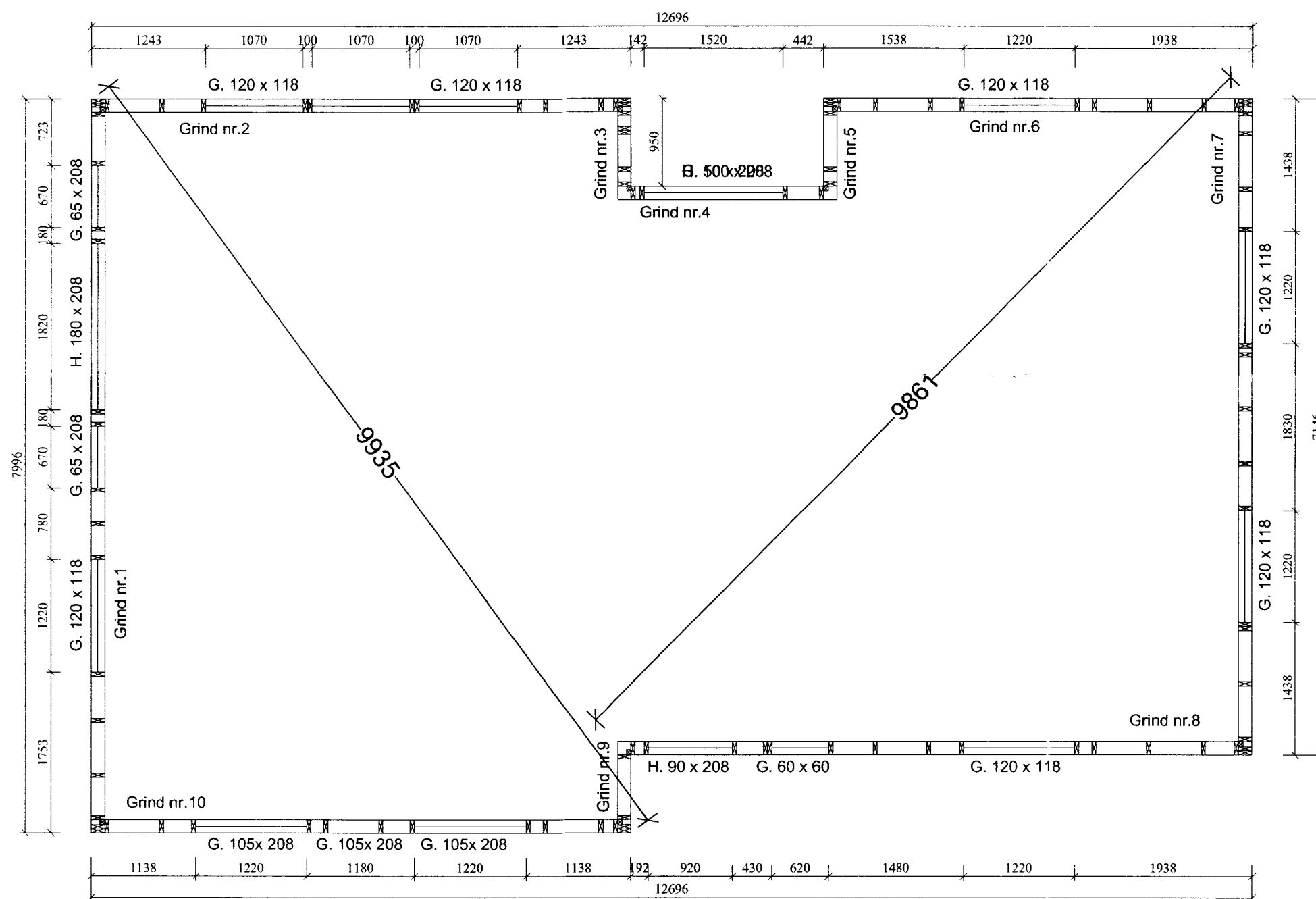
GRUNNMYND 1:50
