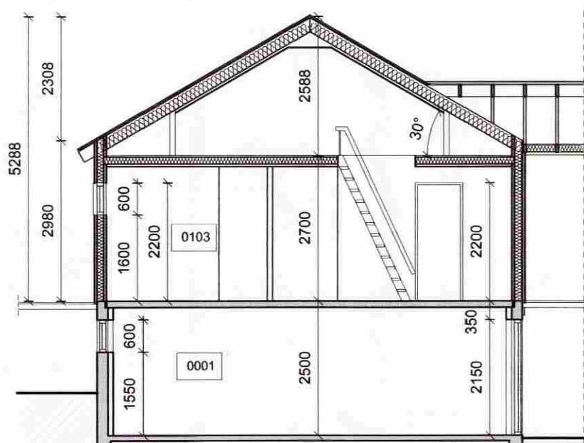
SNID B-B Mkv. 1:100
