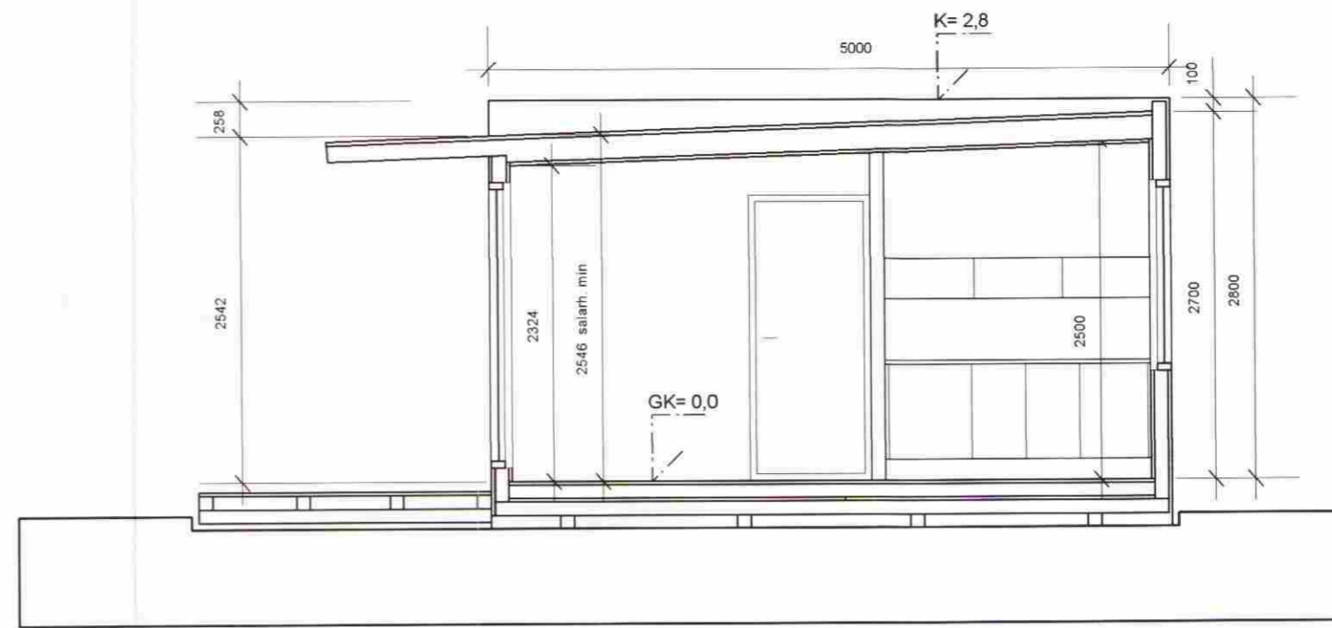
SNEIÐING A-A
