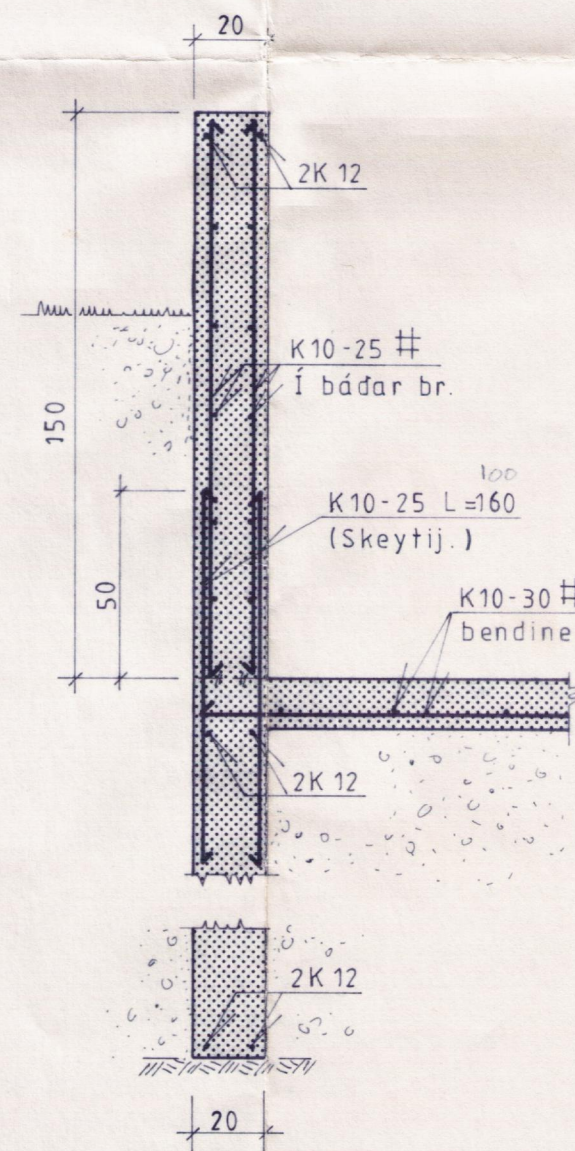
Snid V1-V1 M=1:20
