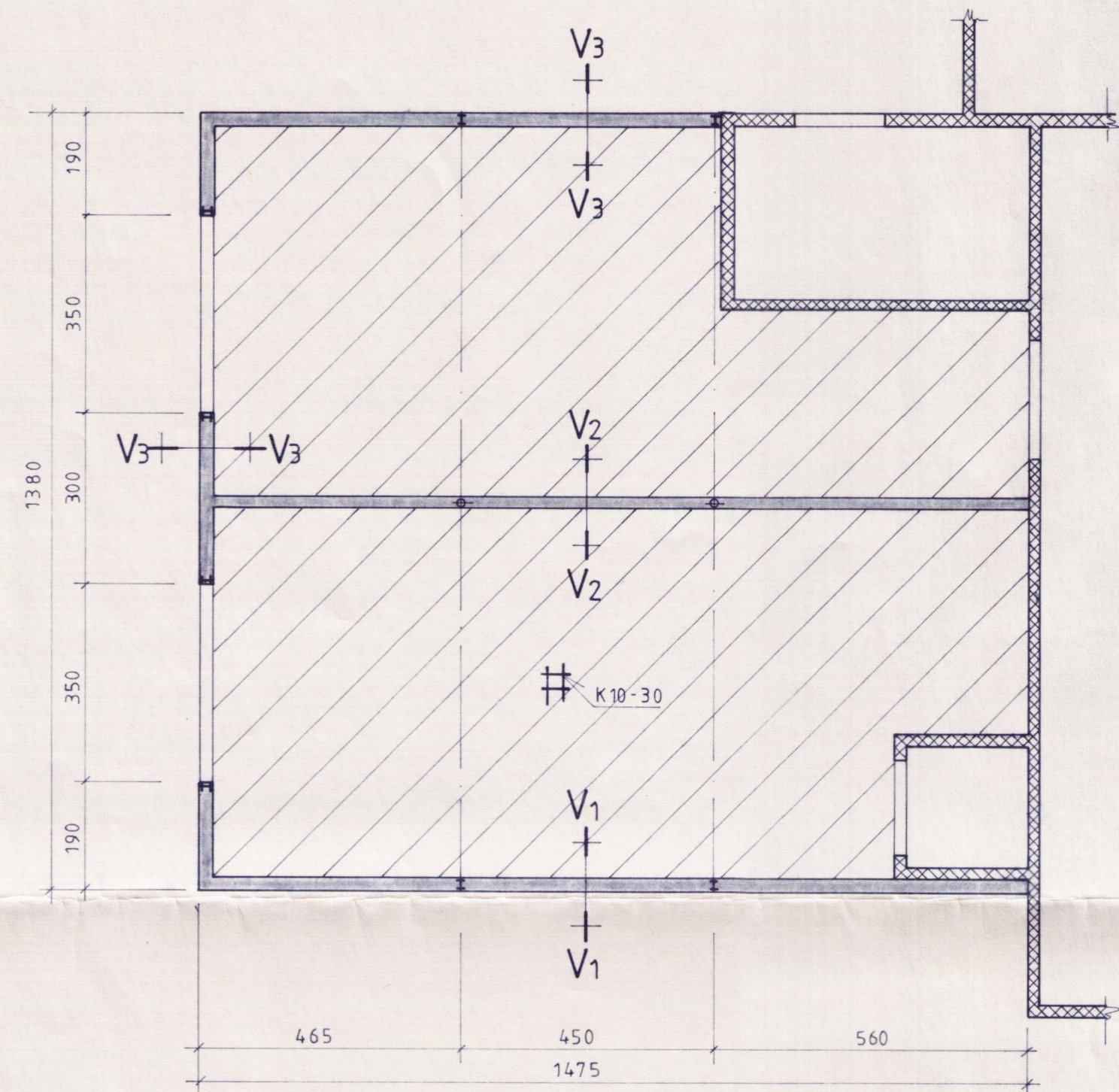
Grunnmynd M=1:100
