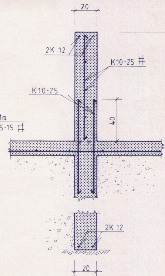
Snid V2-V2 M=1:20
