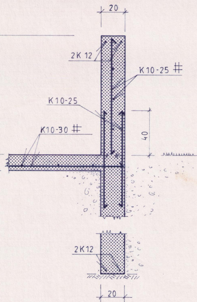
Snid V3-V3 M=1:20
