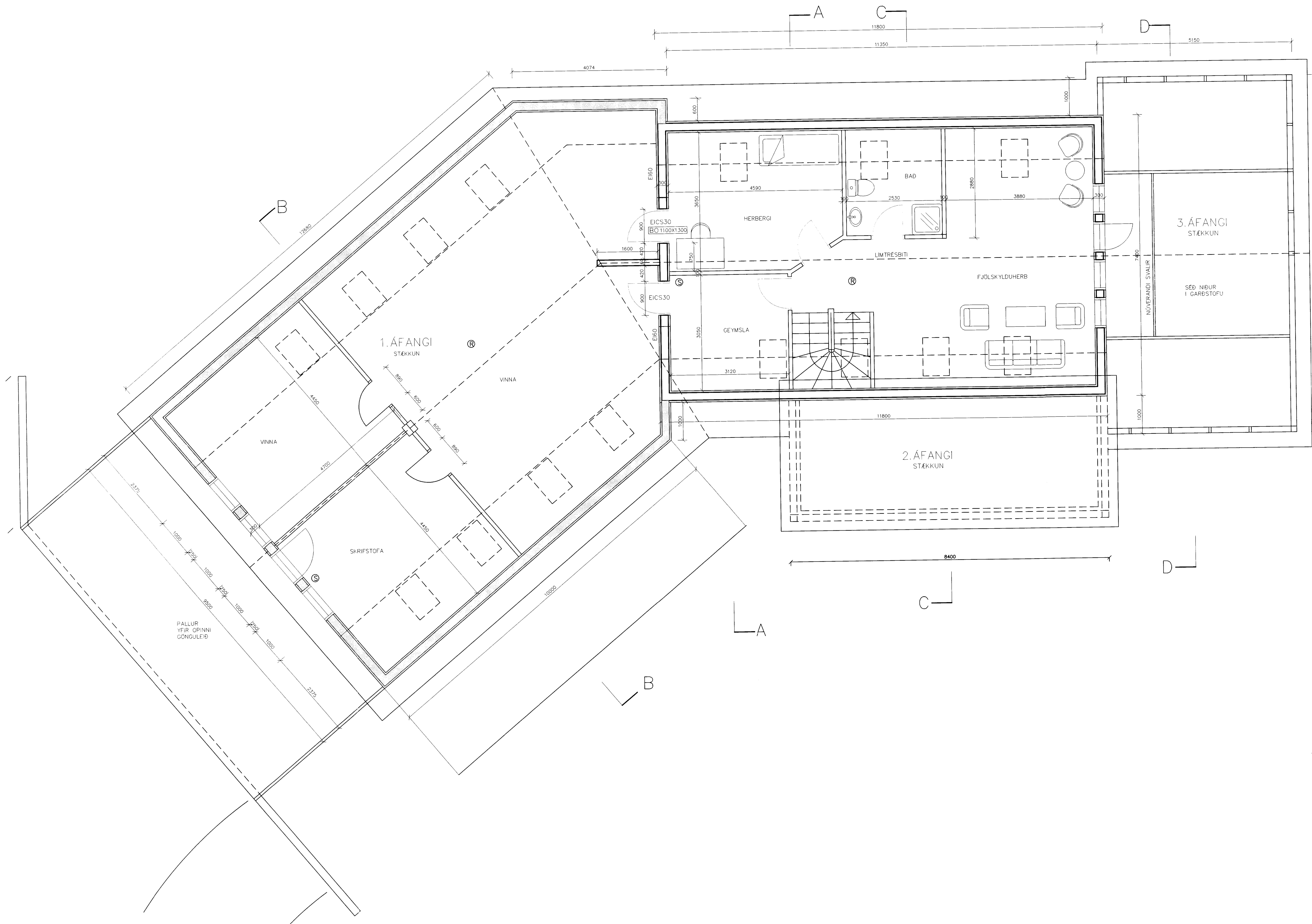
GRUNNMYND 2.. HÆÐ MKV 1:50
