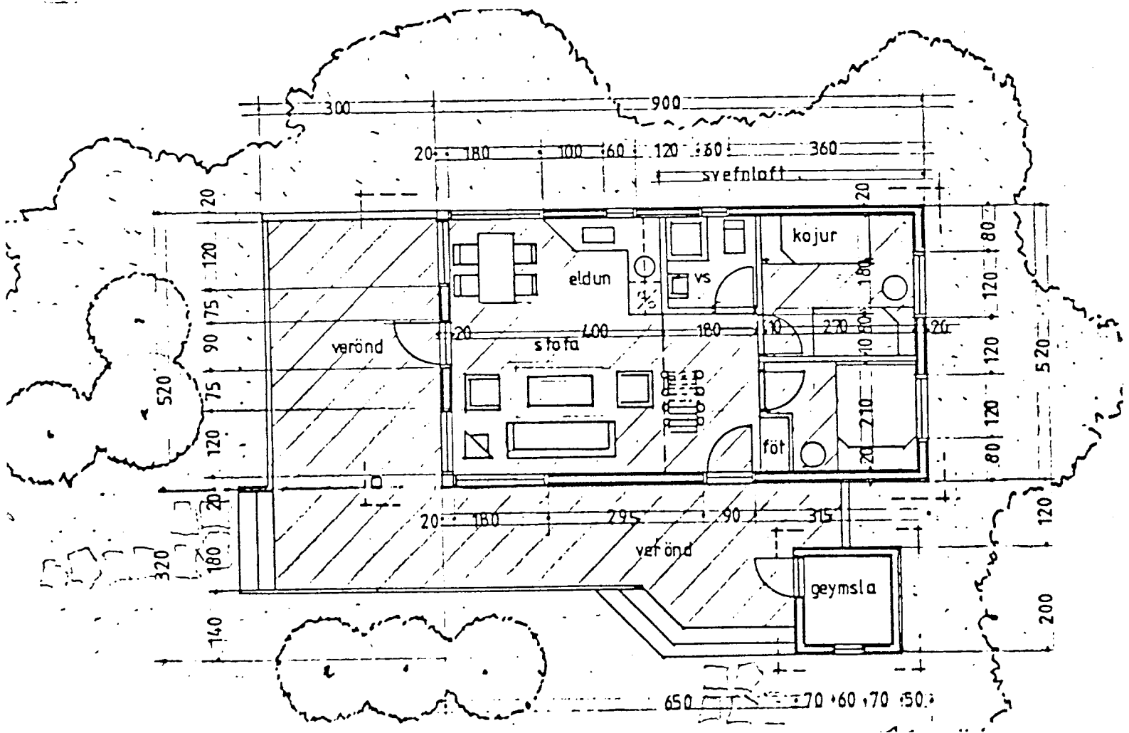
SUMARHÚS 468 m 2
