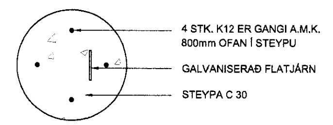
UNDIRSTÖÐUR GRUNNMYND Mkv.:1:10
