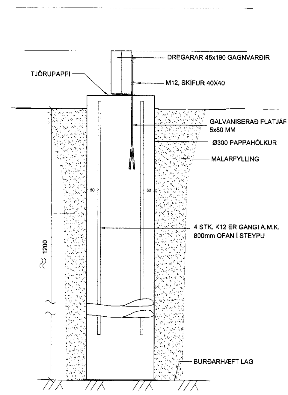
UNDIRSTÖÐUR Mkv.:1:10
