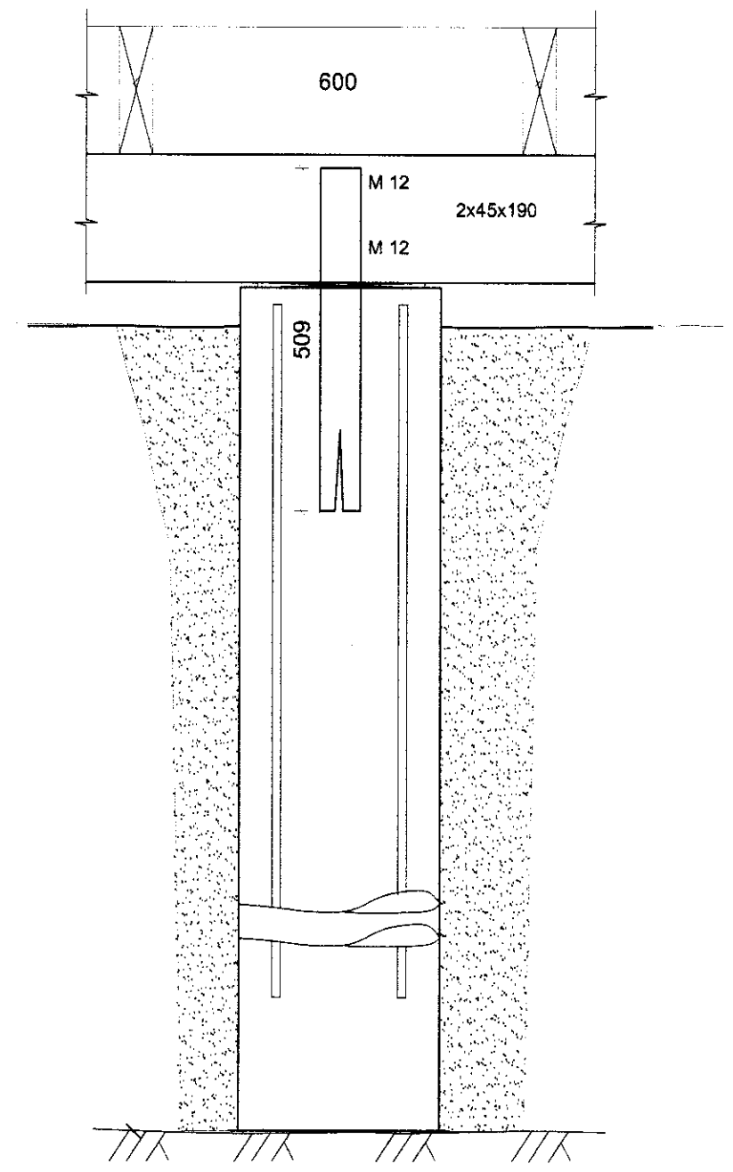
UNDIRSTÖÐUR SNIÐ A Mkv.:1:10
