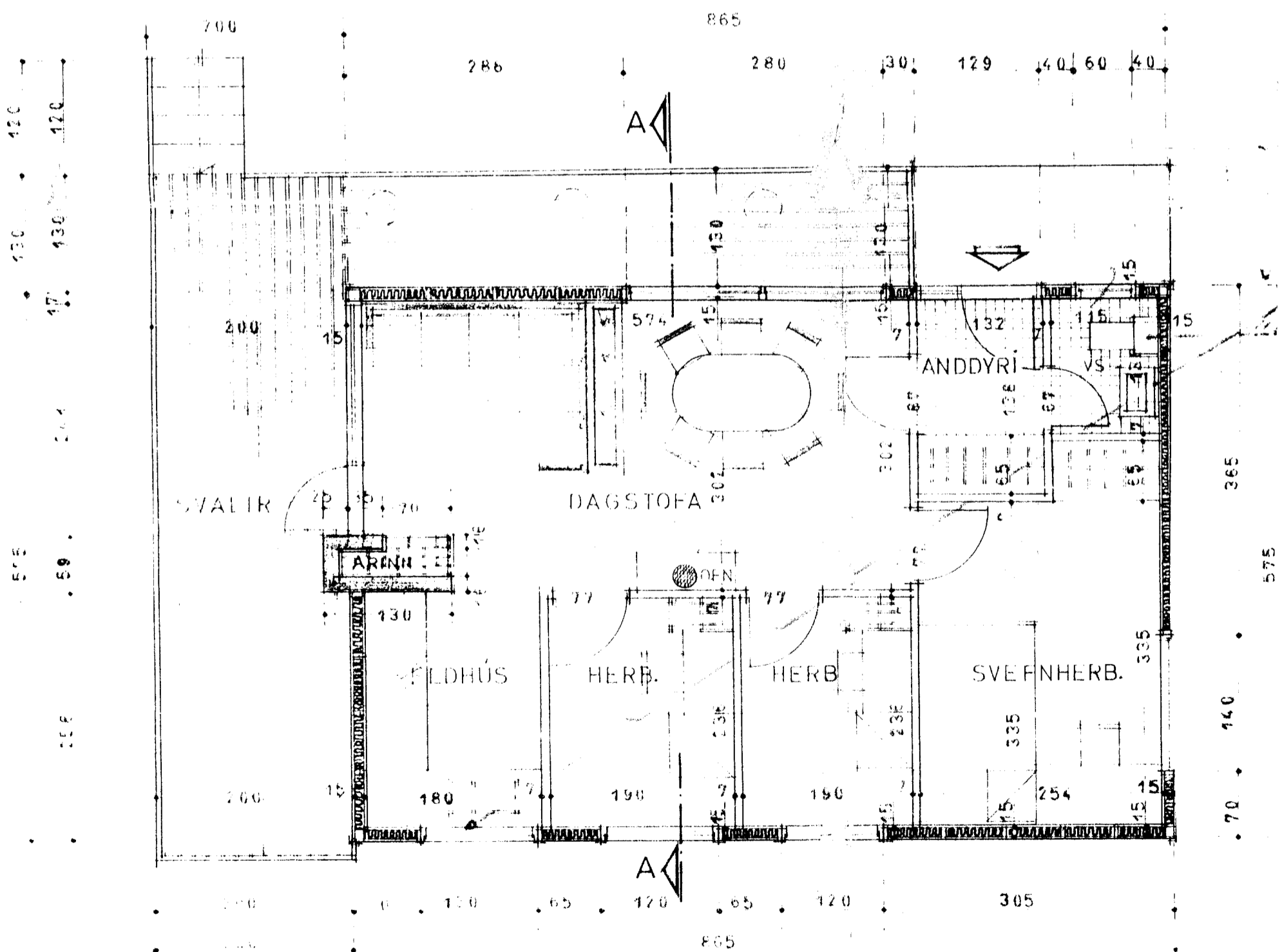
GRUNNMYND M:1:50
