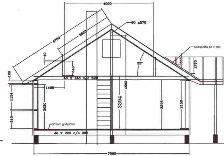
SNÍÐ A-A
